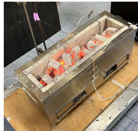
⑦最高温度付近での燃烧状態（オガ炭（白）） 2
