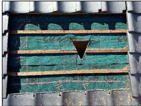
【母屋、垂木位置の明示】
