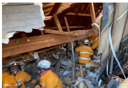
【パイプジャックによる簡易ショアリソク】
