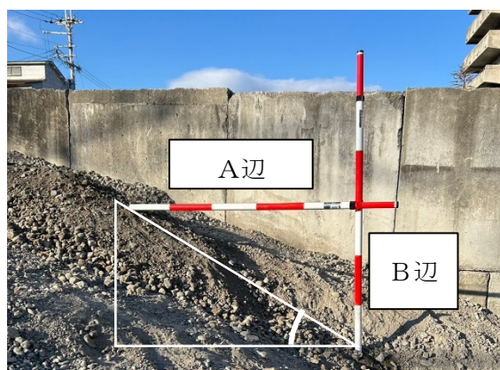
[各辺長と斜面角度の関係図]
