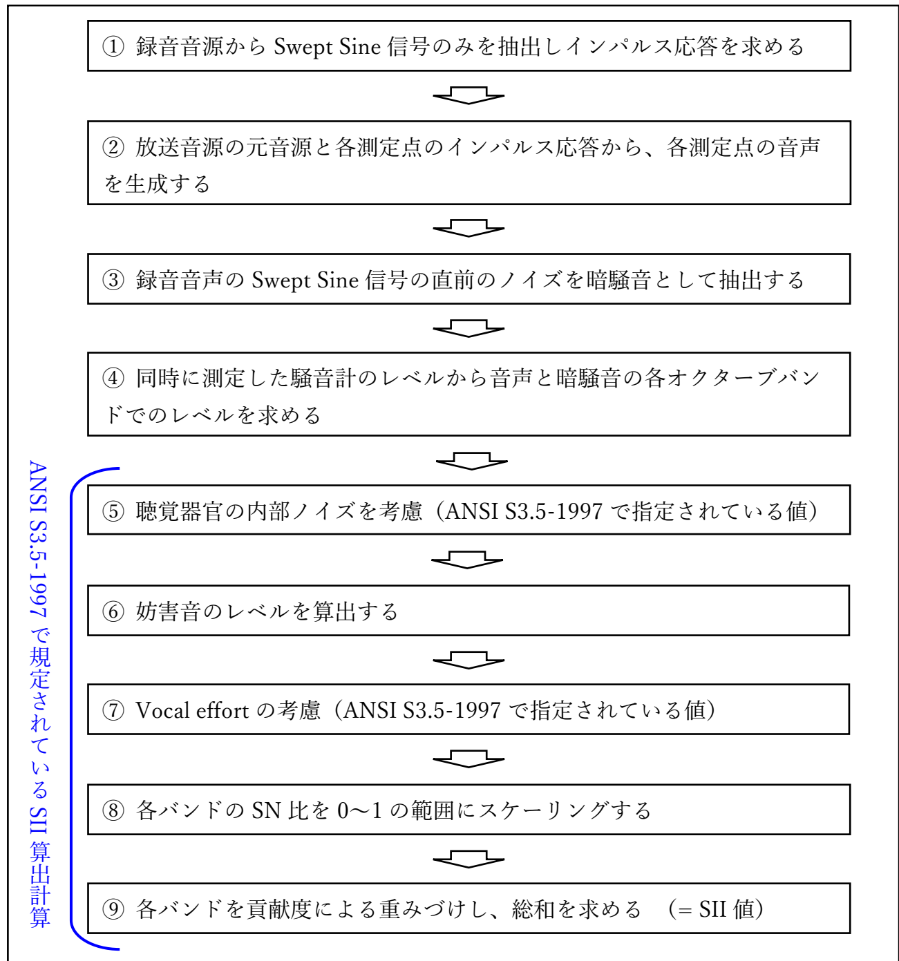
図 115 Swept-Sine 信号からの SII 計算手順
