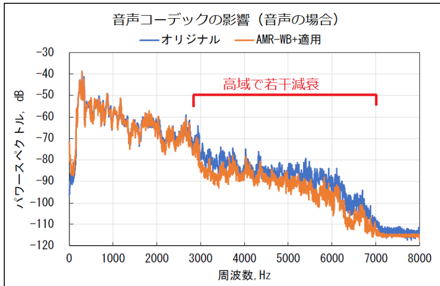
図 12 音声コーデックによる高域減衰の例
