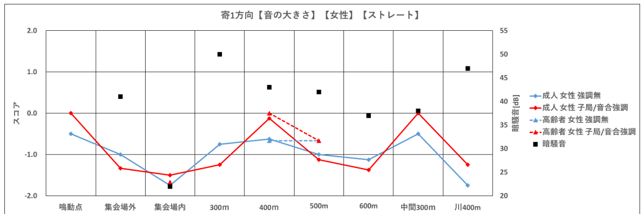
図 209 ストレートホーン【音の大きさ、寄自然休養村、女性】
