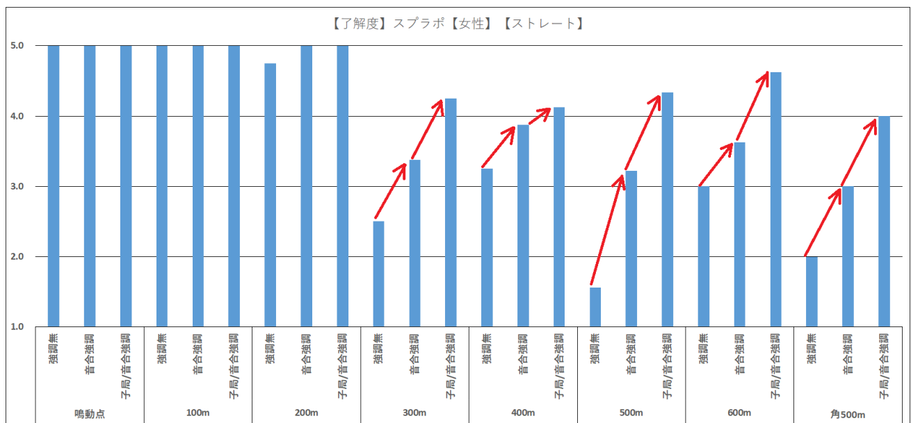
図 22 了解度【スプラボ、話者女性、ストレートホーン】
