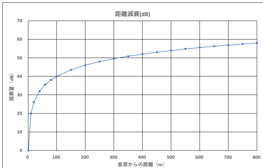
図 307 距離減衰
