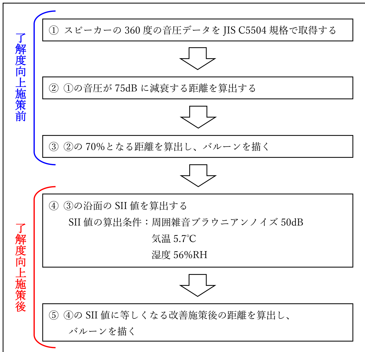
図 298 了解度バルーンの計算手順
