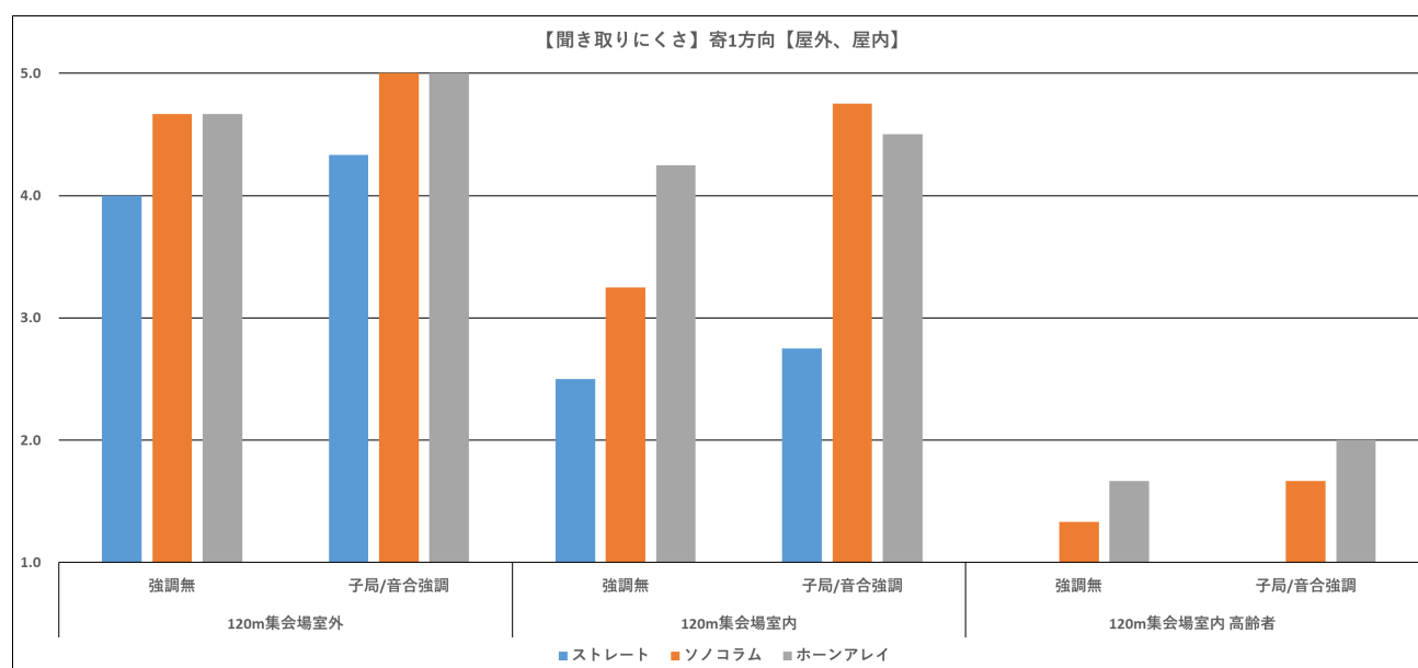
図 240 屋外と屋内【聞き取りにくさ、寄自然休養村、女性、全スピーカー】
