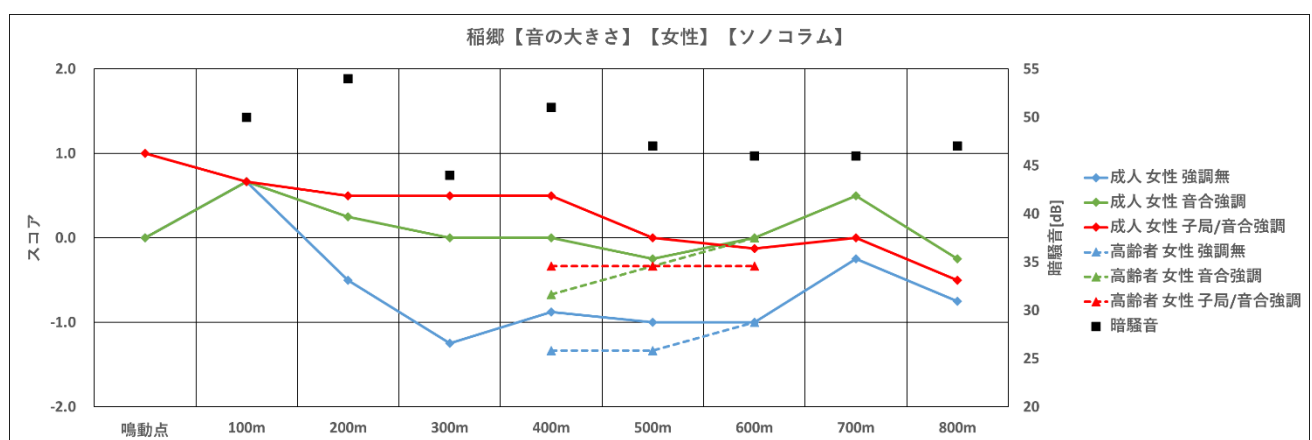
図 203 ソノコラム【音の大きさ、稲郷町有地、女性】
