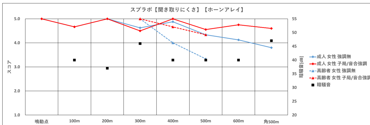
図 168 ホーンアレイ【聞き取りにくさ、スプラボ、女性】
