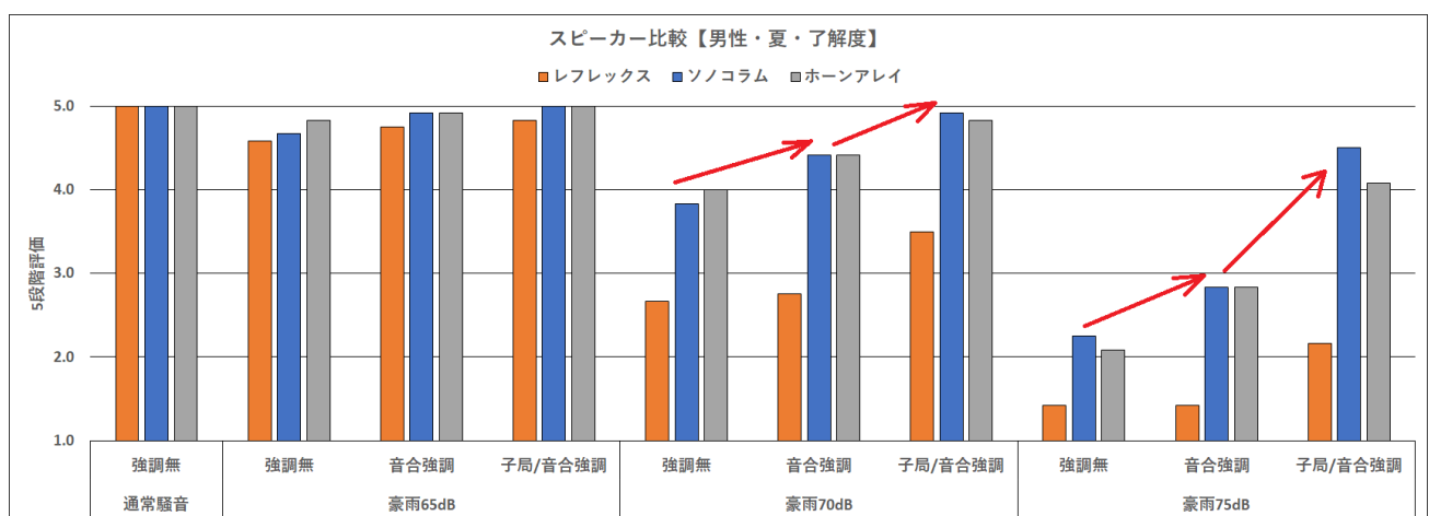
図 15 豪雨下（夏）での了解度改善
