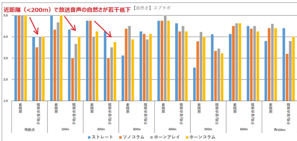
図 317 近距離における周波数強調での自然さ低下例（図 25 引用）
