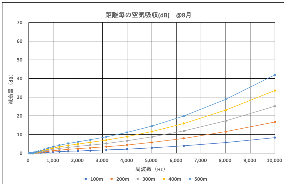
図 306 距離毎の空気吸収による減衰量の試算結果【8月想定】
