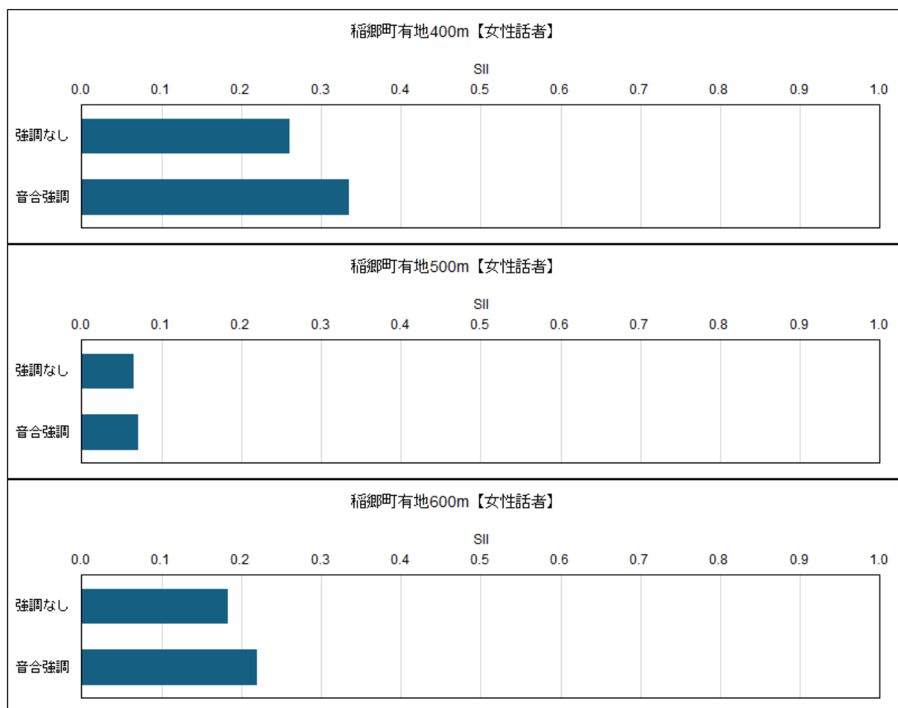
図 118 稲郷町有地 SII
