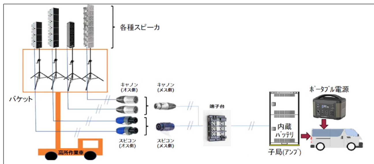
図 146 放送設備
