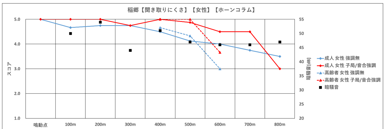
図 174 ホーンコラム【聞き取りにくさ、稲郷町有地、女性】
