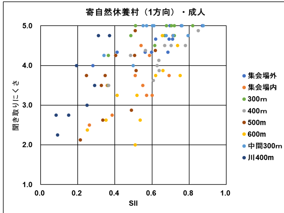
図 291 SII と聞き取りにくさの関係【寄自然休養村 1 方向、成人】
