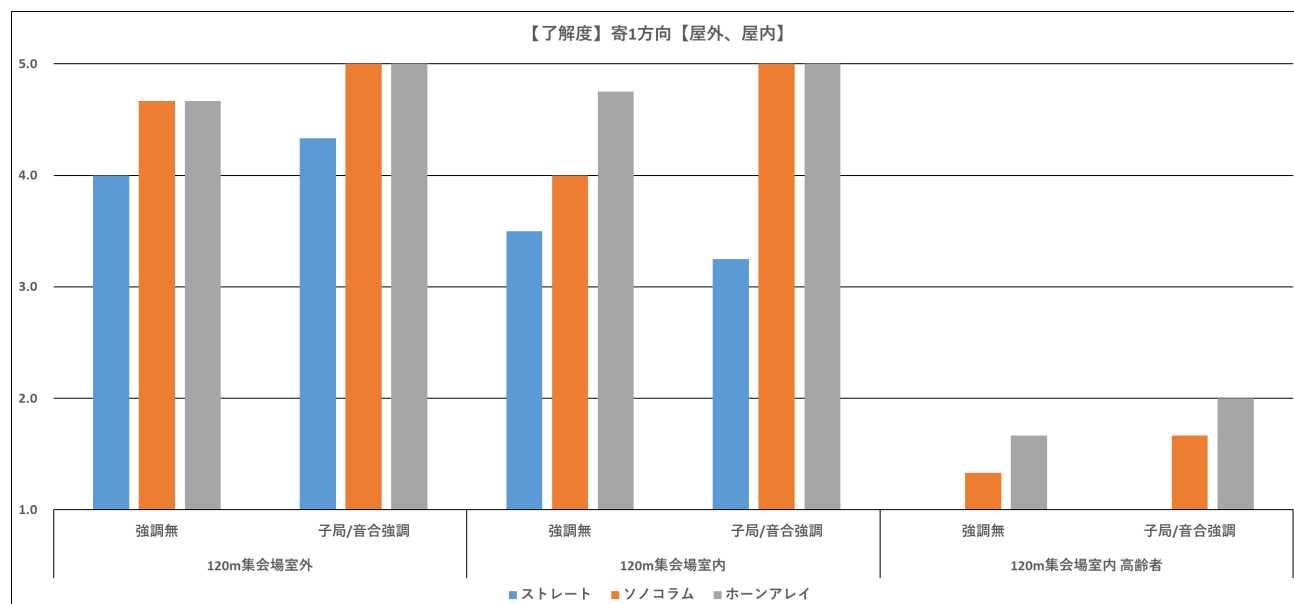
図 239 屋外と屋内【了解度、寄自然休養村、女性、全スピーカー】
