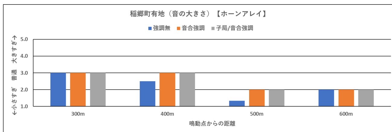
図 134 稲郷町有地（ホーンアレイ）【音の大きさ】
