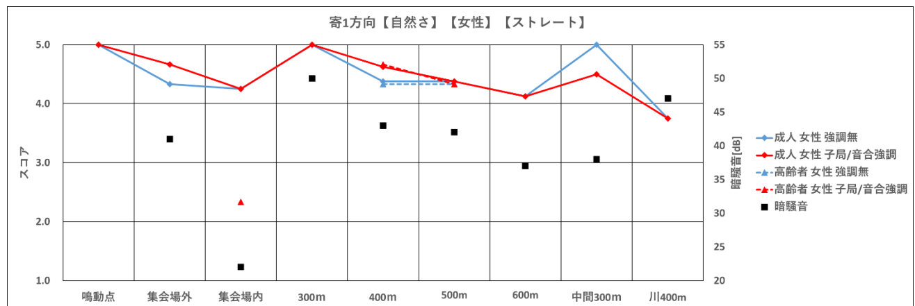
図 190 ストレートホーン【自然さ、寄自然休養村、女性】
