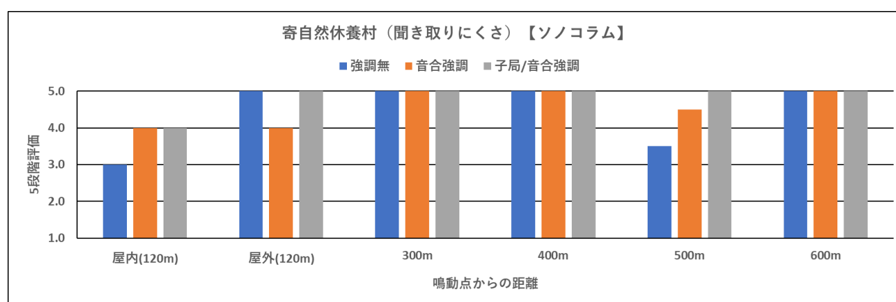
図 132 寄自然休養村（ソノコラム）【聞き取りにくさ】
