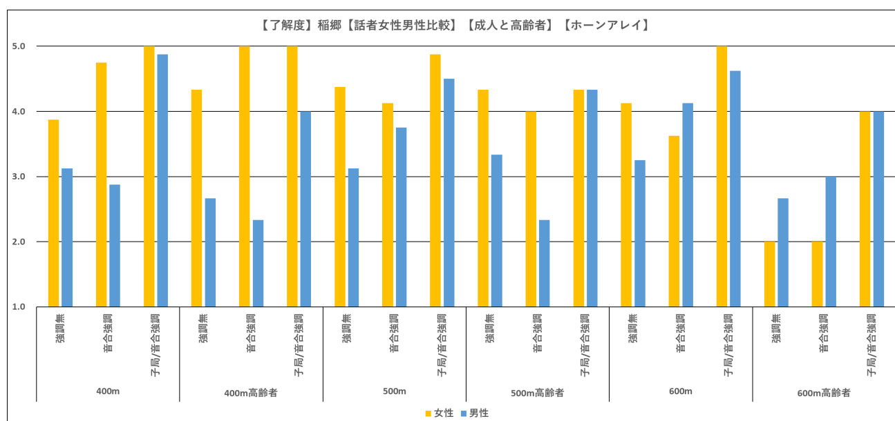
図 233 話者（男女）の違い【了解度、稲郷町有地、成人・高齢者、ホーンアレイ】
