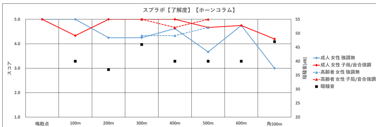
図 155 ホーンコラム【了解度、スプラボ、女性】
