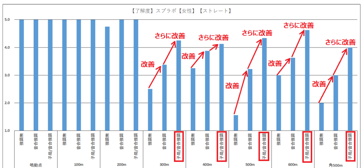
図 316 子局と音声合成の周波数強調併用による了解度改善例（図 22 引用）
