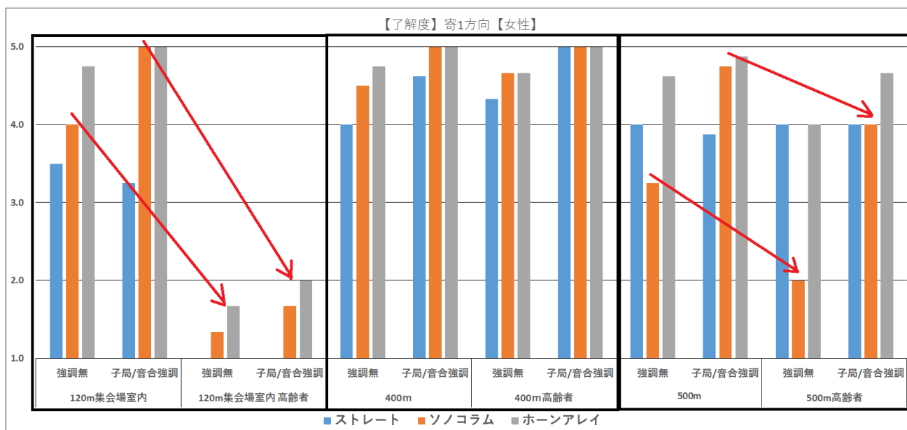
図 32 成人高齢者比較【了解度、寄自然休養村、女性話者】
