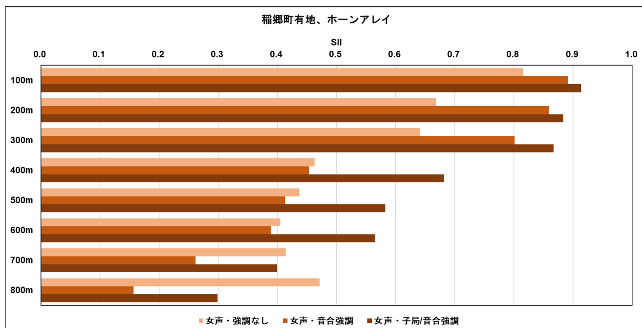
図 276 SII【稲郷町有地、女性、ホーンアレイ】
