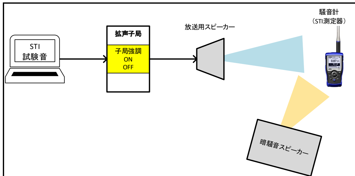
図 49 STI 測定系
