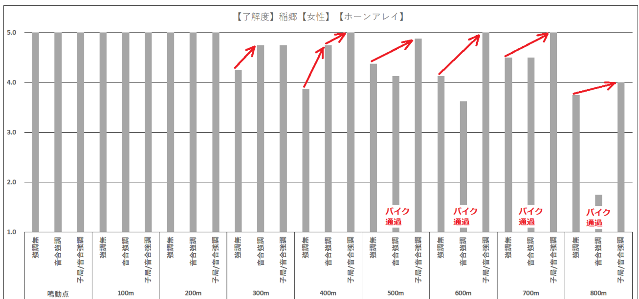
図 24 了解度【寄自然休養村、話者女性、ホーンアレイ】
