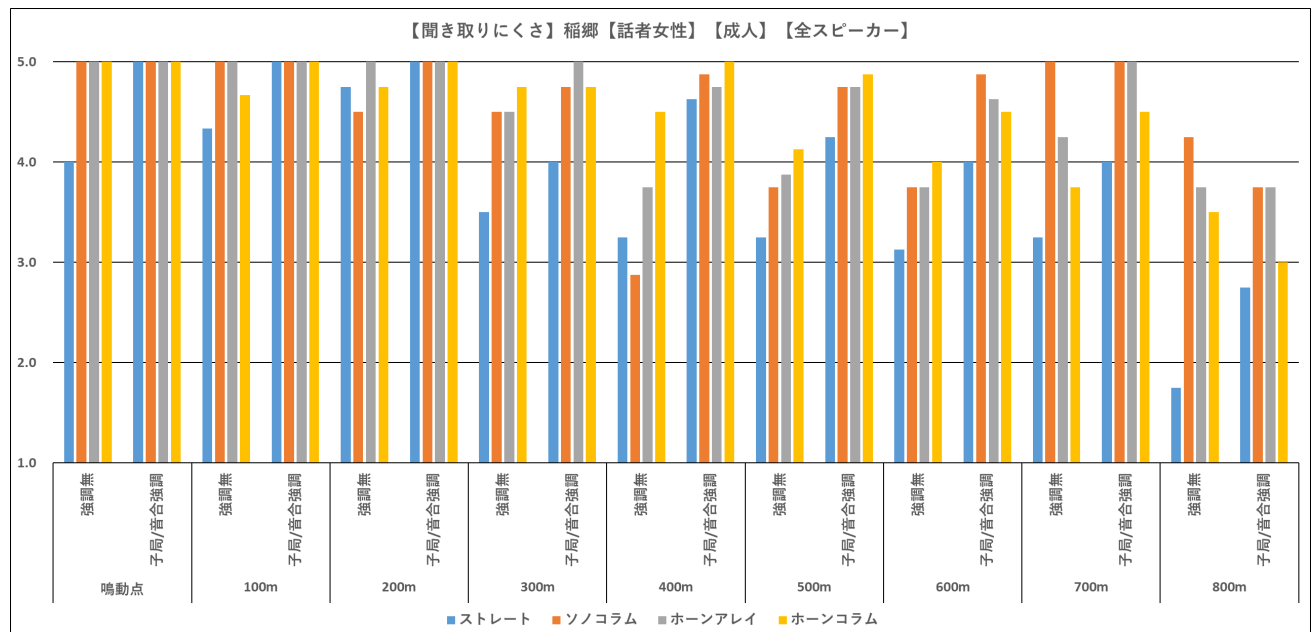
図 170 スピーカー比較【聞き取りにくさ、稲郷町有地、女性、成人、全スピーカー】
