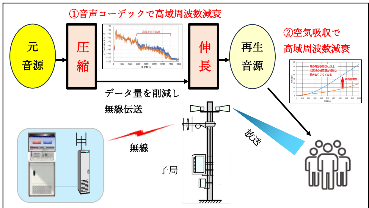
図 315 高域周波数の減衰要因
