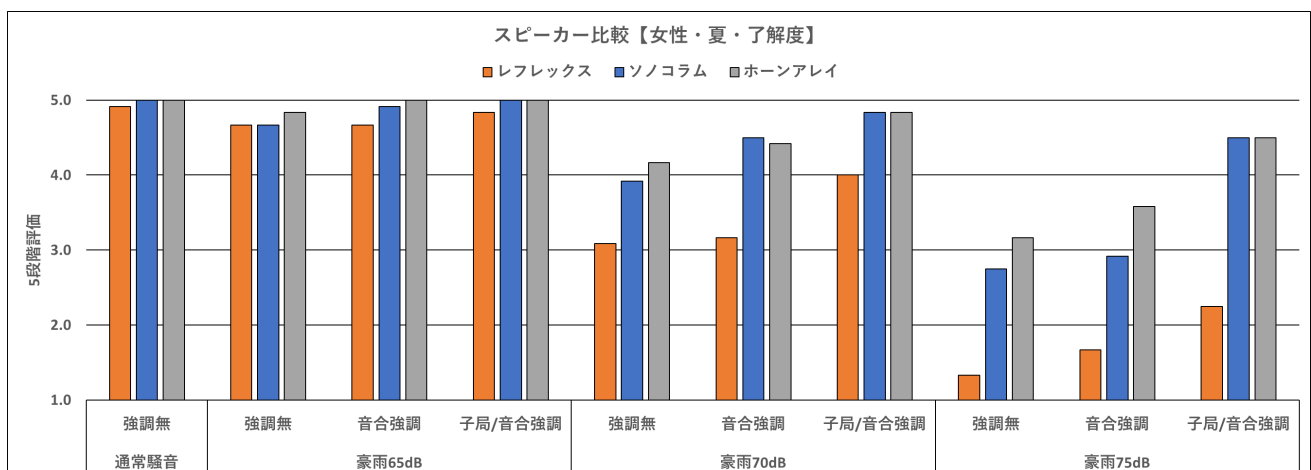
図 56 スピーカー比較【女性・夏・了解度・豪雨】
