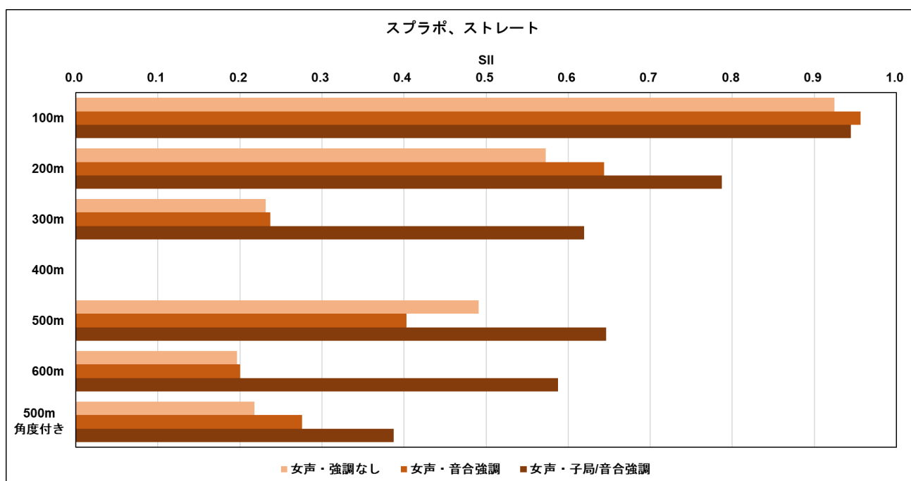
図 269 SII【スプラボ、女性、ストレートホーン】
