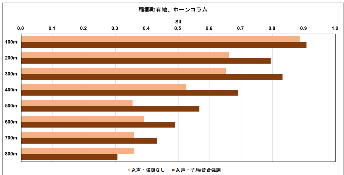
図 278 SII【稲郷町有地、女性、ホーンコラム】
