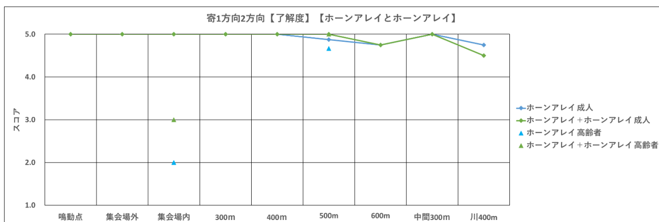
図 248 一方向二方向比較【了解度、寄自然休養村、女性、成人・高齢者、ホーンアレイ】
