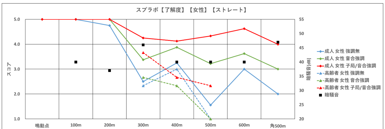
図 152 ストレートホーン【了解度、スプラボ、女性】
