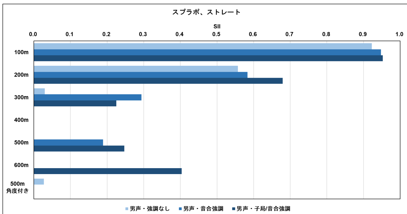
図 270 SII【スプラボ、男性、ストレートホーン】
