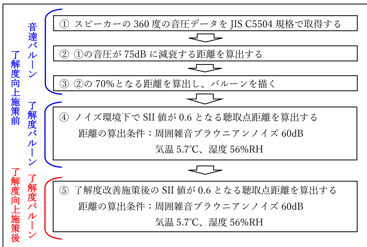
図 300 ノイズ環境下の了解度バルーンの計算手順
