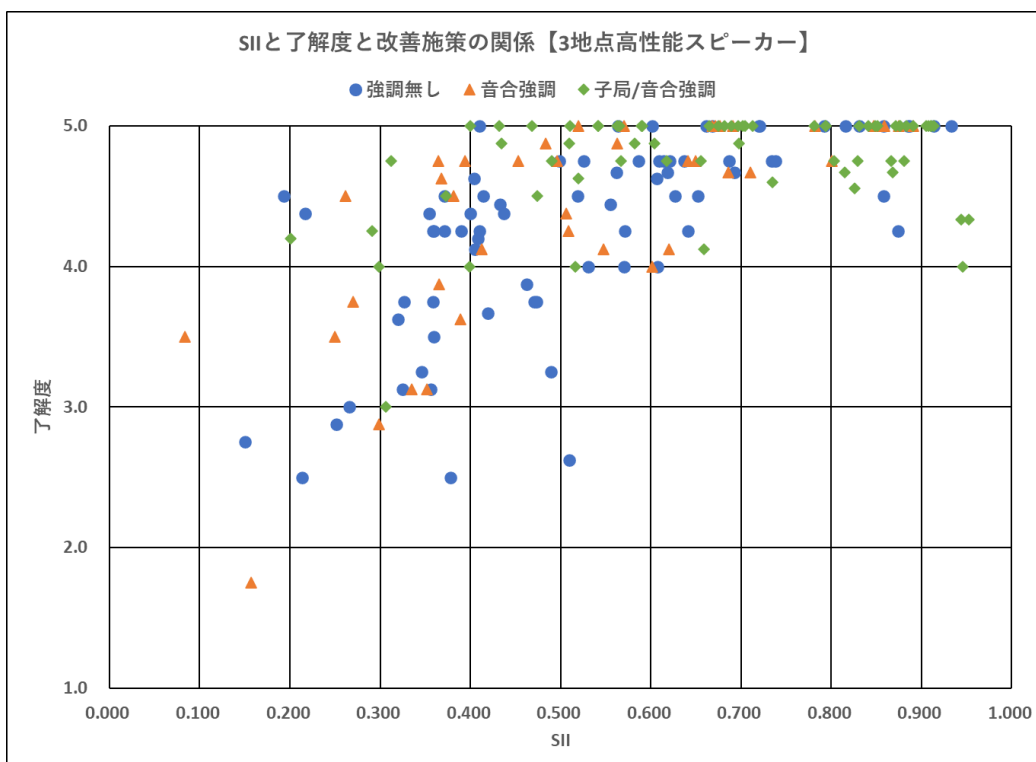
図 286 SII と了解度と改善施策の関係【高性能スピーカー】
