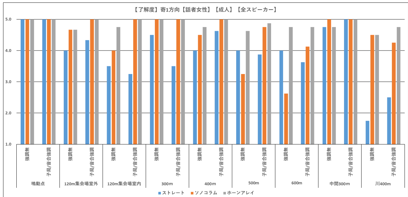
図 161 スピーカー比較【了解度、寄自然休養村、女性、成人、全スピーカー】
