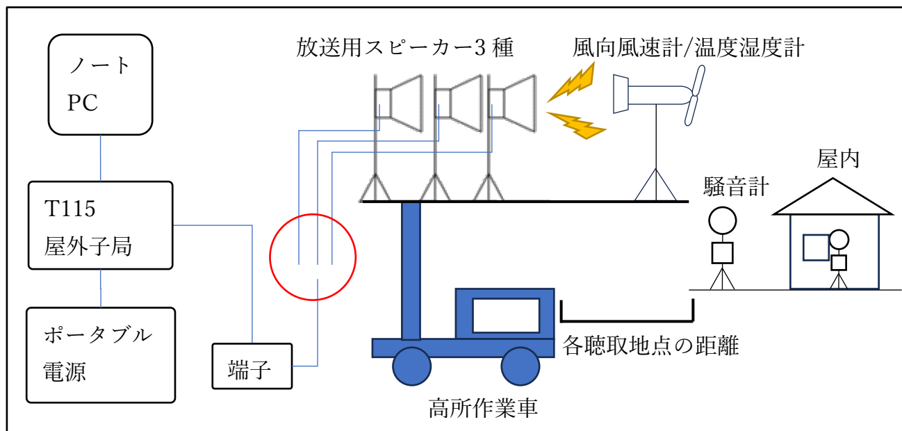
図 113 第二回実証実験機器構成
