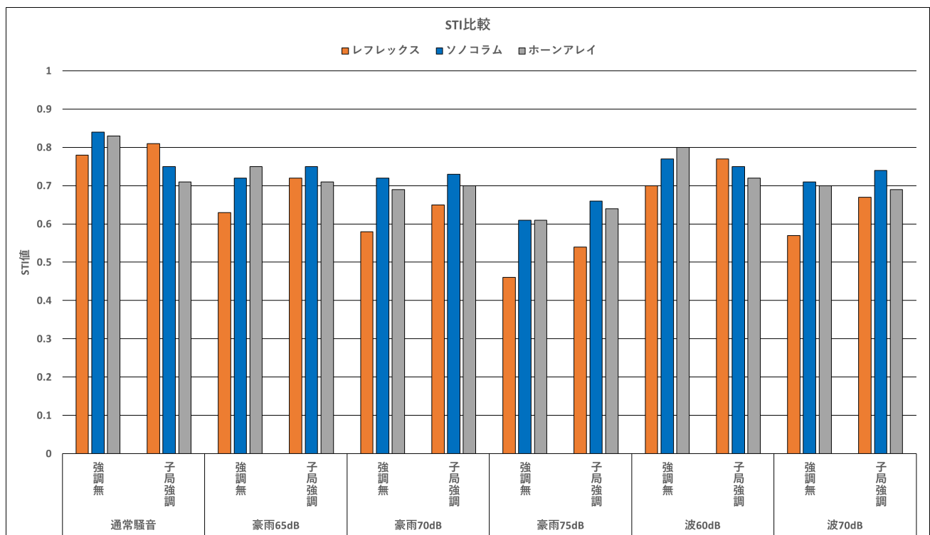
図 106 STI 測定結果
