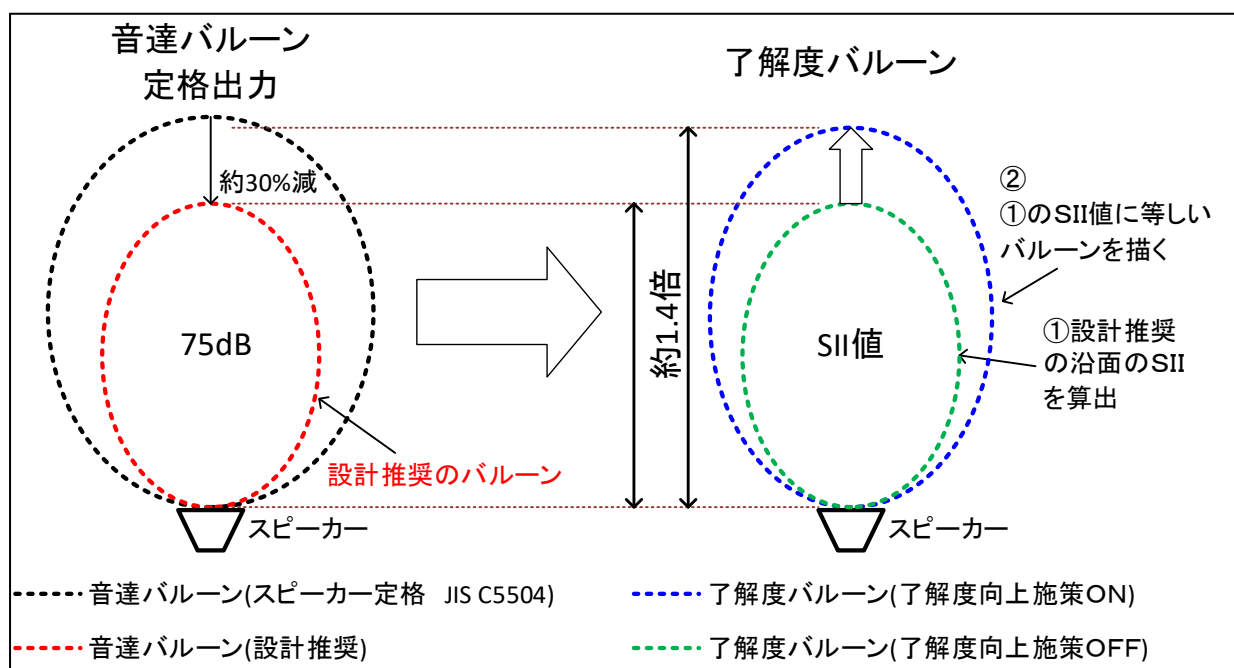
図 38 検討①了解度バルーンイメージ
