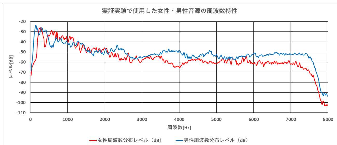
図 148 音声放送（女性・男性）の周波数特性
