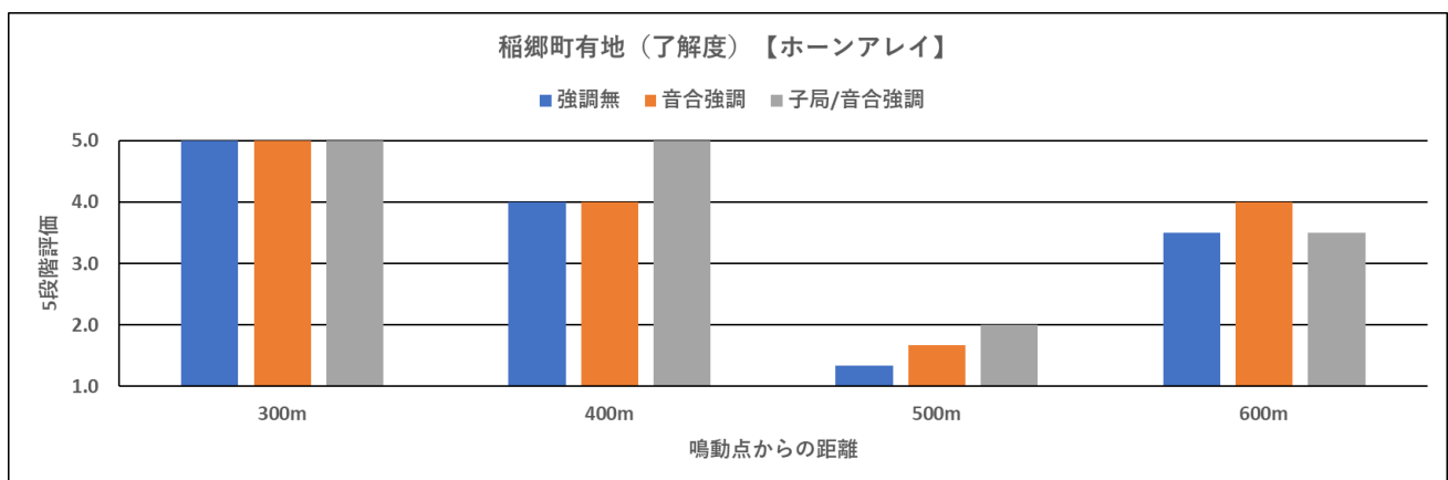
図 125 稲郷町有地（ホーンアレイ）【了解度】
