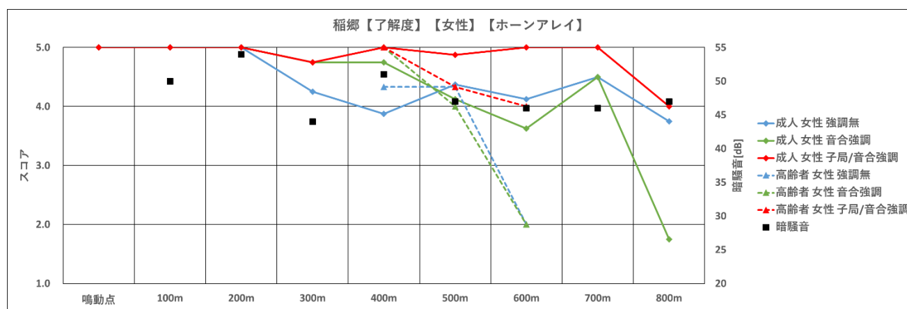
図 159 ホーンアレイ【了解度、稲郷町有地、女性】
