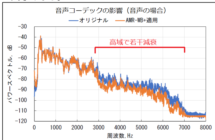
図 313 音声コーデックによる高域周波数減衰例（図 12 再掲）
