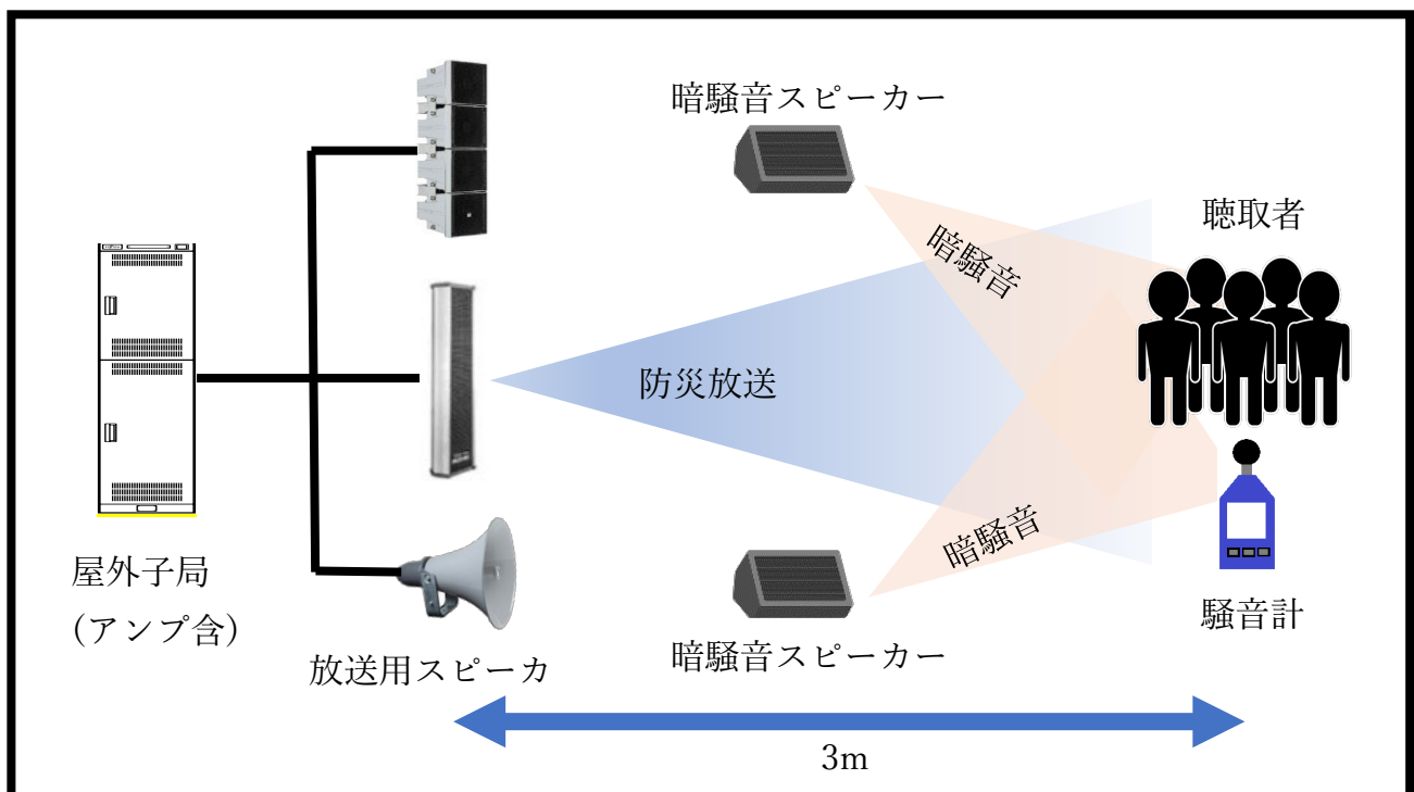
図 42 第一回実証実験試験環境イメージ
