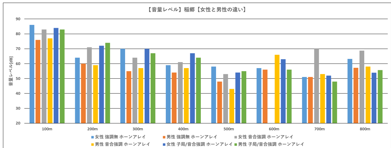
図 237 話者（男女）の違い【音量レベル、稲郷町有地、ホーンアレイ】
