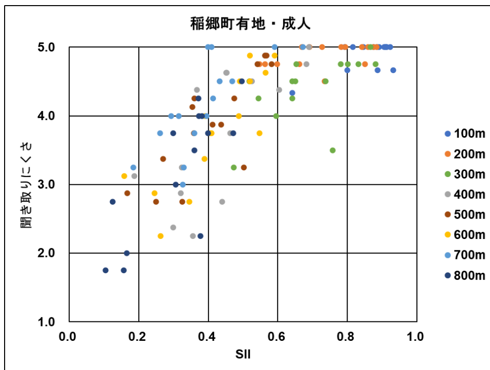
図 289 SII と聞き取りにくさの関係【稲郷町有地、成人】
