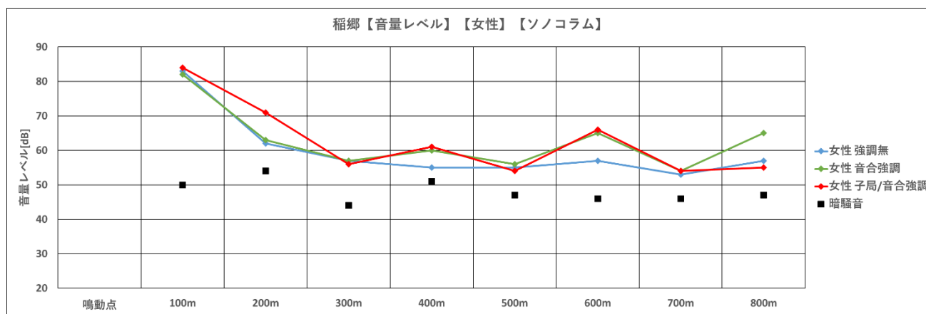
図 204 ソノコラム【音量レベル、稲郷町有地、女性】
