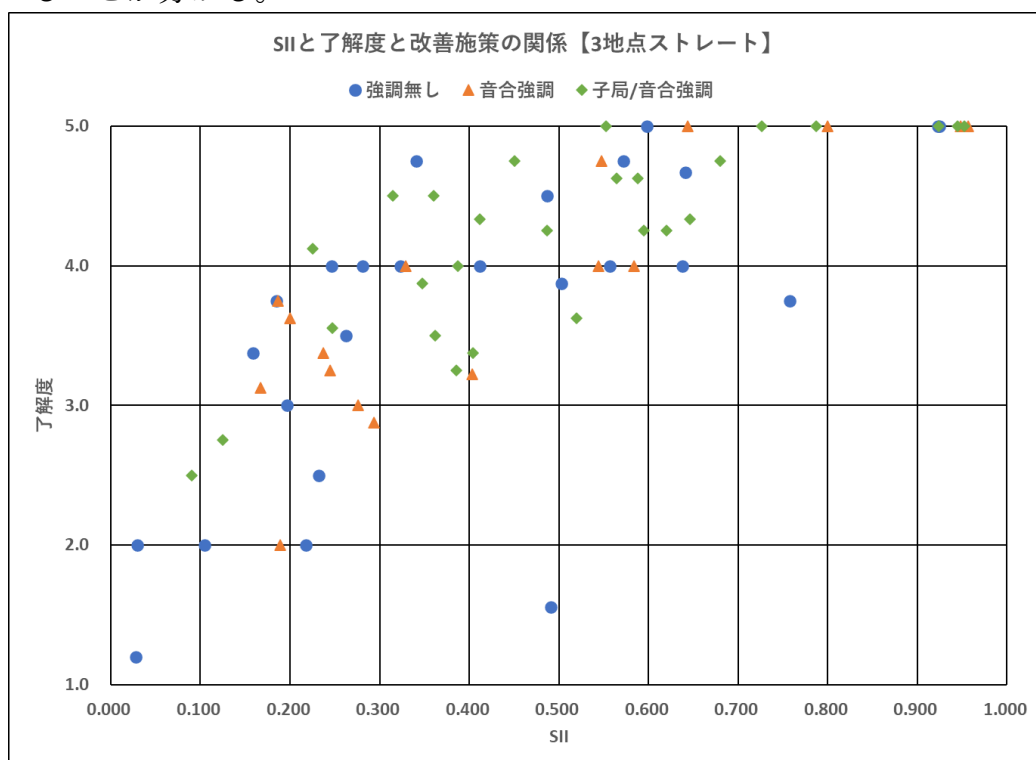
図 285 SII と了解度と改善施策の関係【ストレートホーン】
