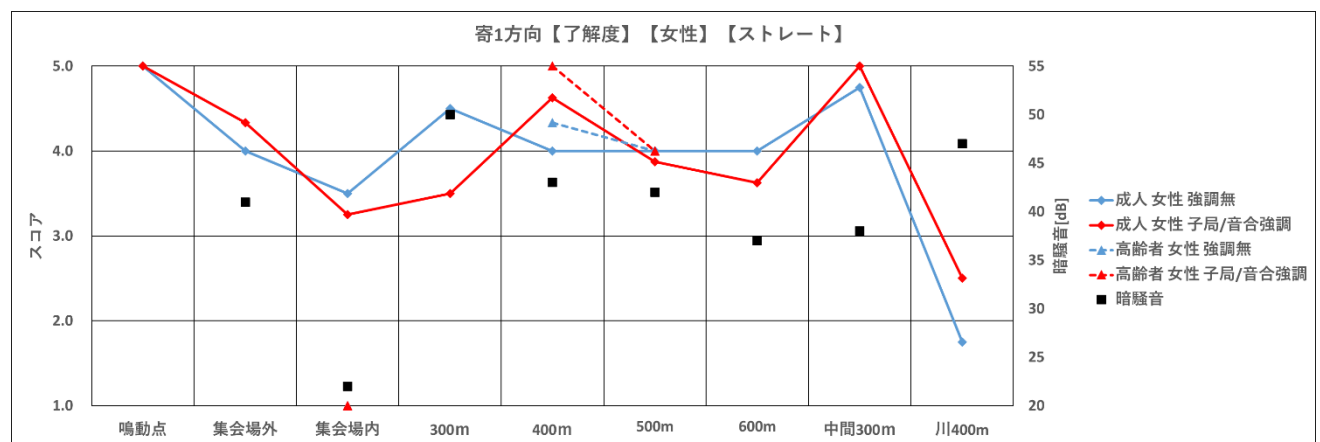
図 162 ストレートホーン【了解度、寄自然休養村、女性】
