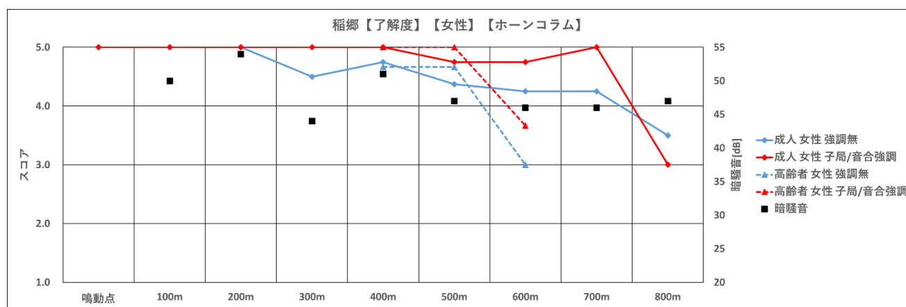
図 160 ホーンコラム【了解度、稲郷町有地、女性】
