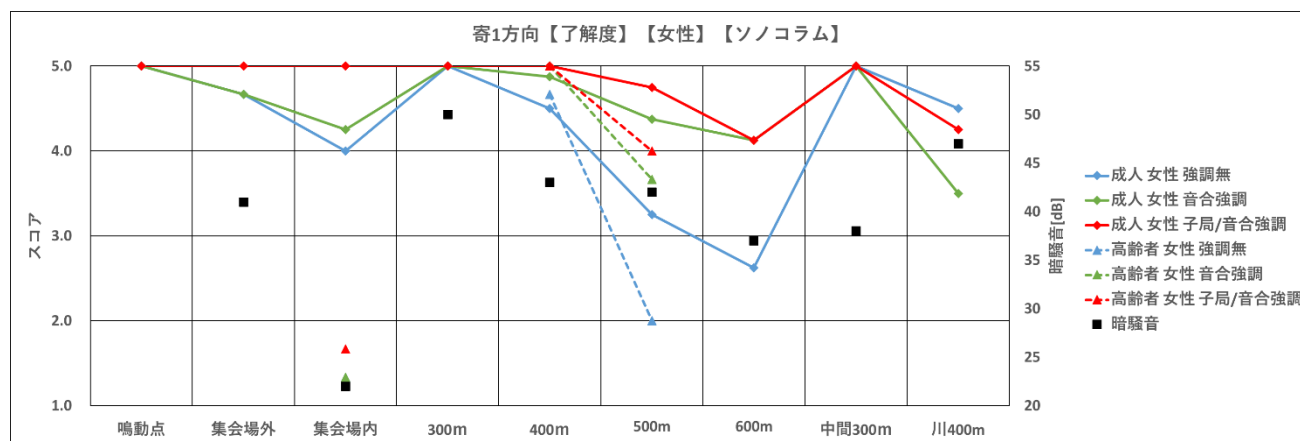
図 163 ソノコラム【了解度、寄自然休養村、女性】
