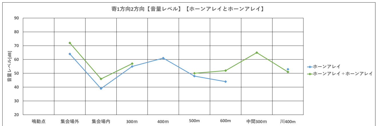
図 265 一方向二方向比較【音量レベル、寄自然休養村、女性、成人・高齢者、ホーンアレイ】
