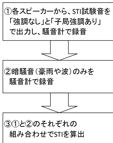
図 50 STI 測定フロー
