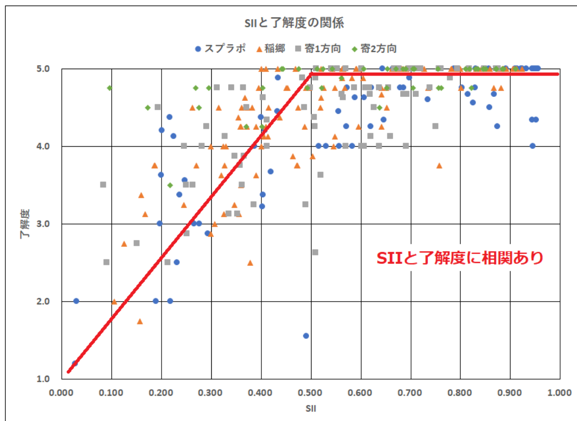
図 37 SII と了解度の関係
