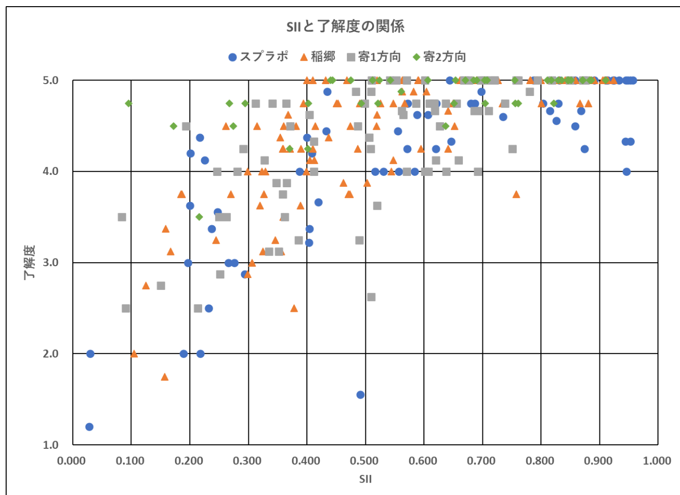
図 284 SII と了解度の関係
