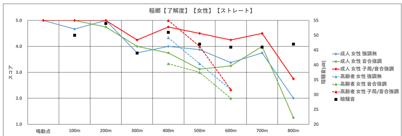
図 157 ストレートホーン【了解度、稲郷町有地、女性】
