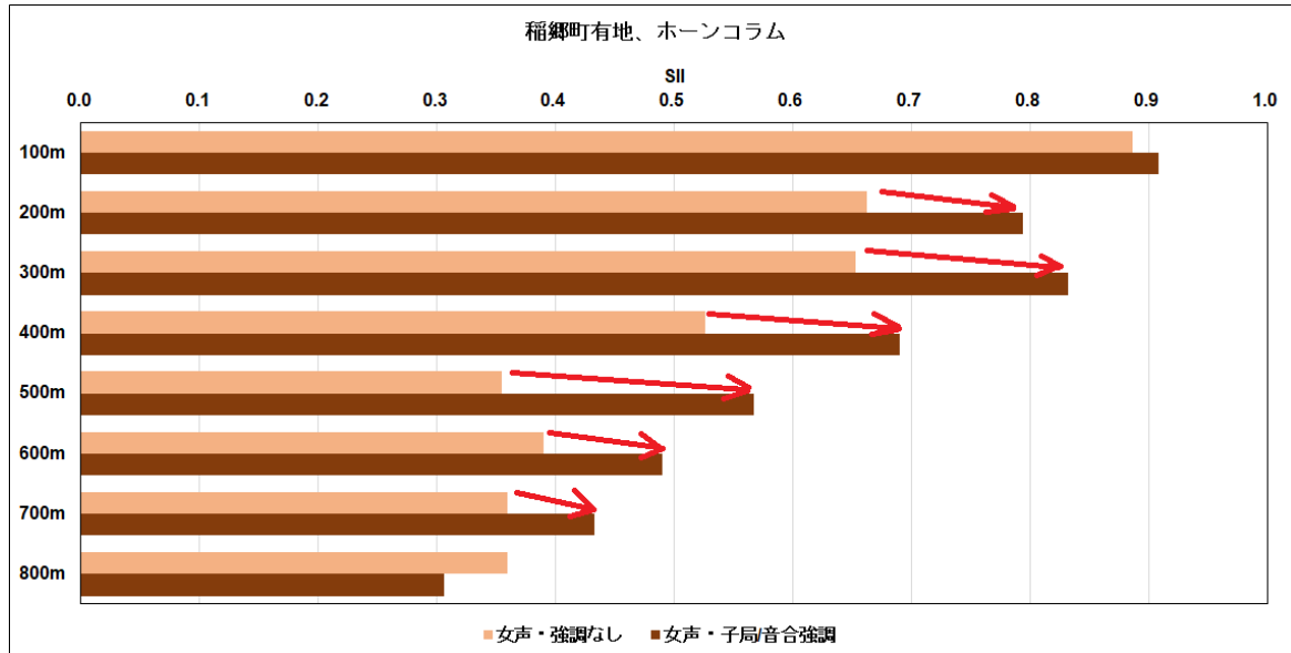
図 35 SII の改善例（稲郷町有地、ホーンコラム）
