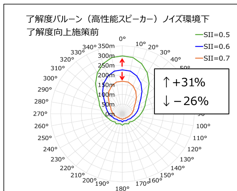
図 304 高性能スピーカーの SII と了解度バルーンの関係
