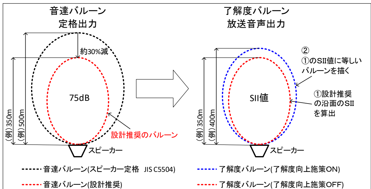
図 297 音達バルーンの机上検討イメージ
