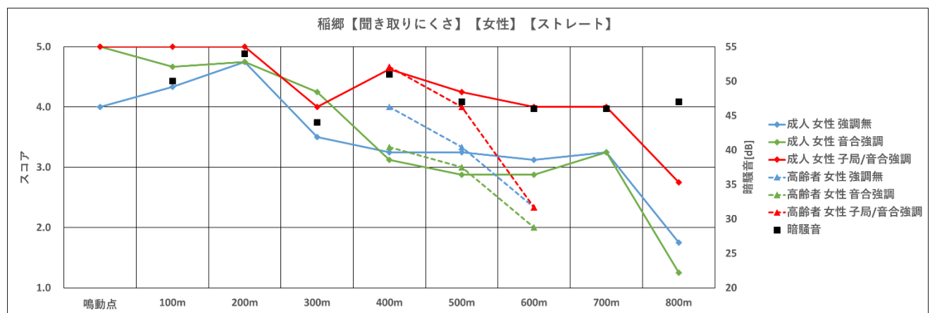
図 171 ストレートホーン【聞き取りにくさ、稲郷町有地、女性】
