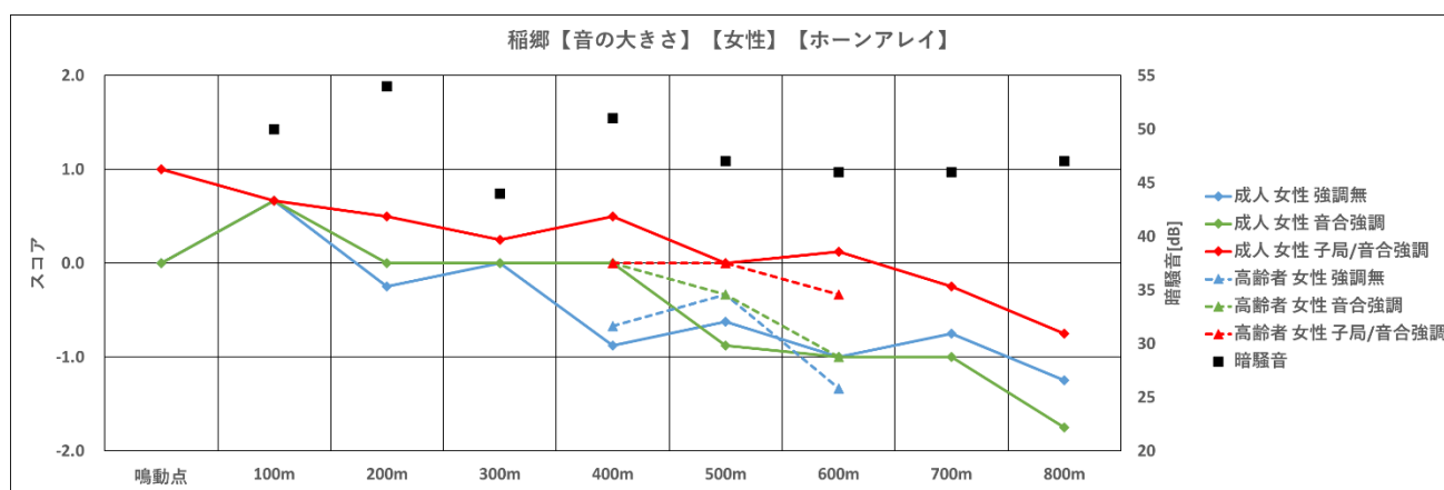
図 205 ホーンアレイ【音の大きさ、稲郷町有地、女性】
