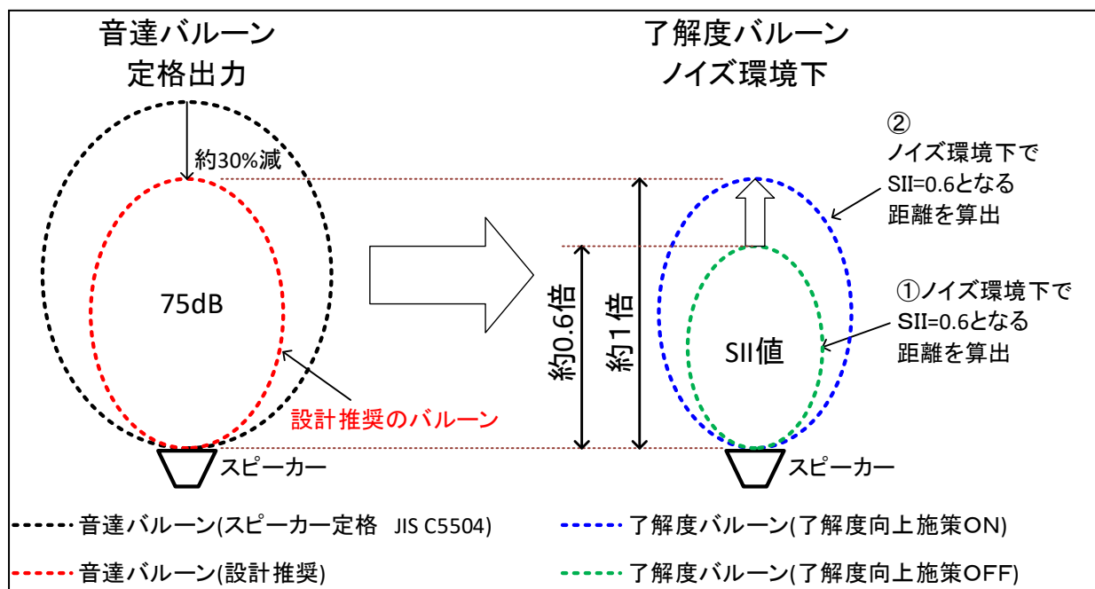
図 39 検討②ノイズ環境下の了解度バルーンイメージ
