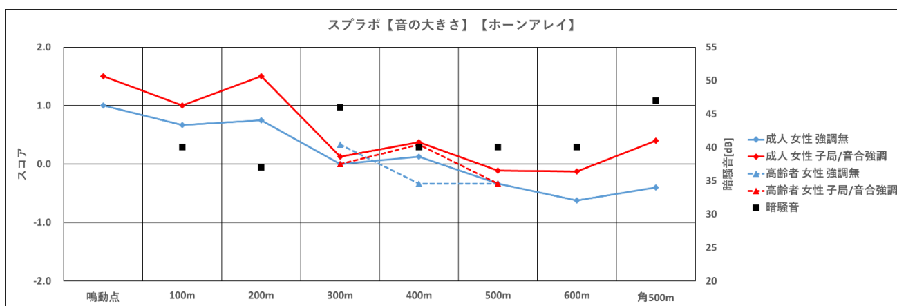
図 197 ホーンアレイ【音の大きさ、スプラボ、女性】
