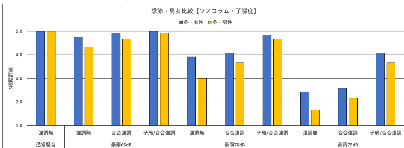
図 73 話者（男女）比較【ソノコラム・冬・了解度・豪雨】
