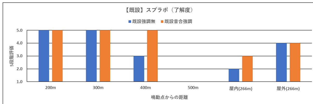
図 136 既設操作卓での音合強調の効果【了解度】
