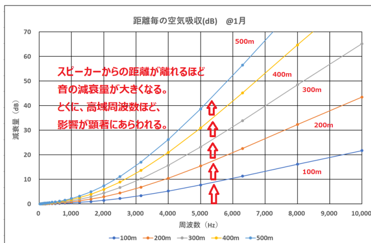
図 314 空気吸収による高域周波数減衰例（図 305 引用）
