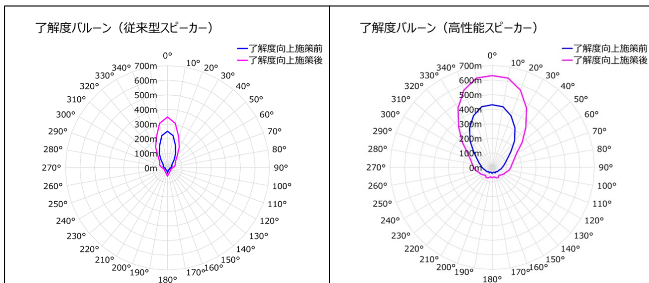
図 299 了解度バルーンの計算例
