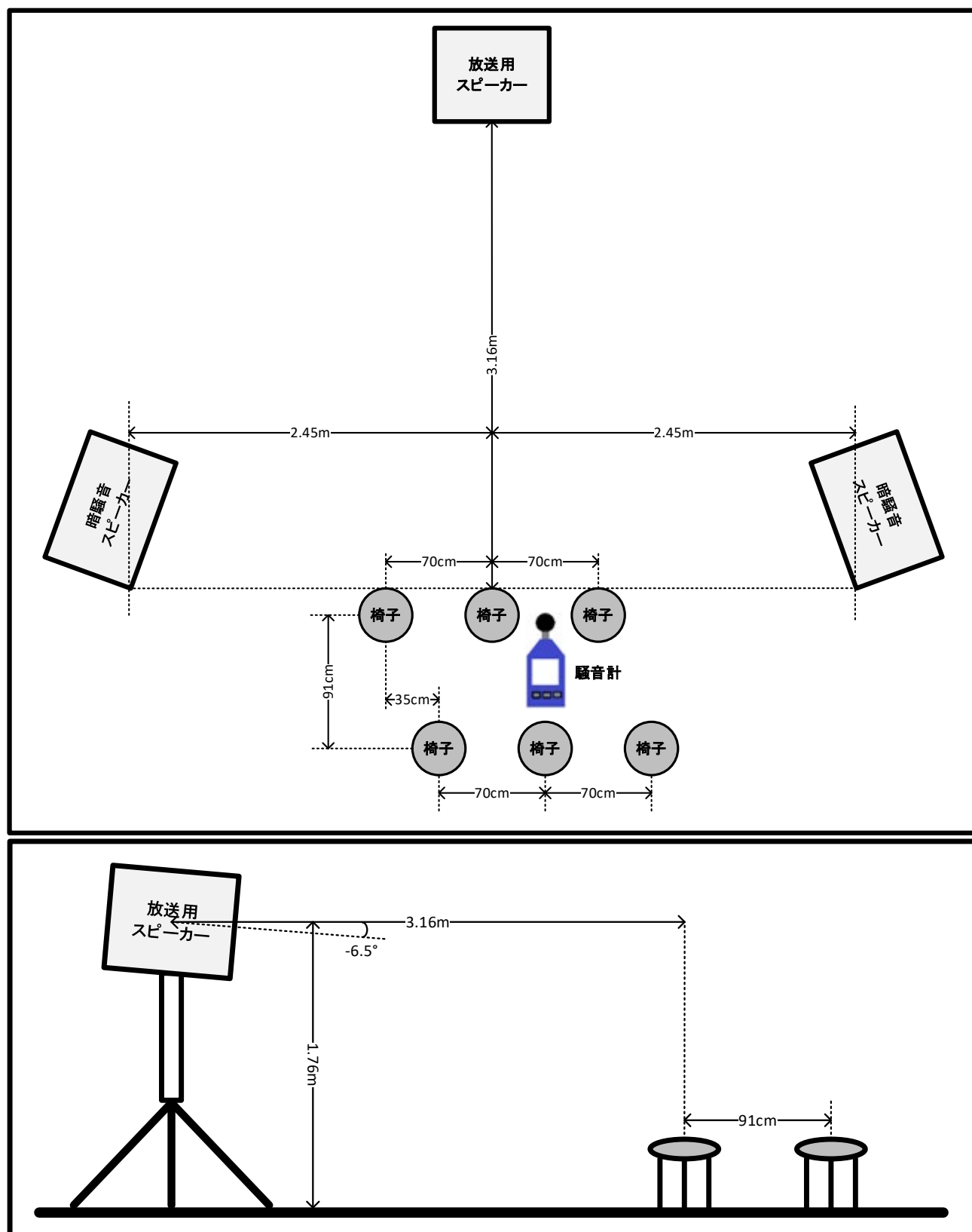
図 46 機器セッティング
