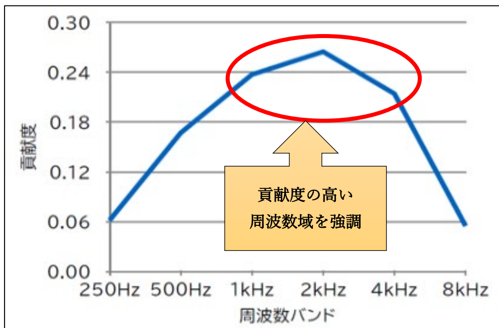
図 10 周波数バンドと SII への貢献度の関係
