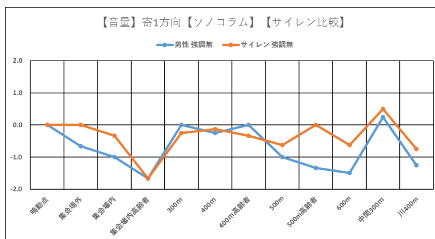
図 268 音声と電子サイレン【音の大きさ、寄自然休養村、ソノコラム】
