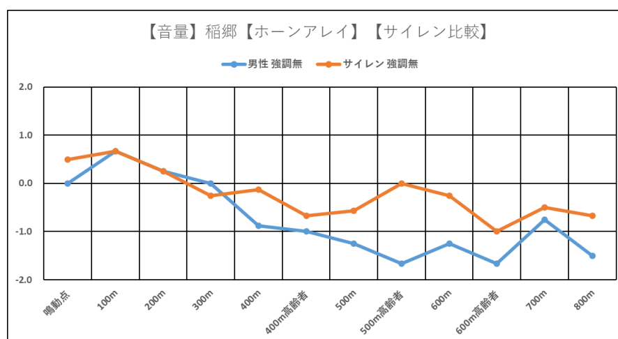
図 267 音声と電子サイレン【音の大きさ、稲郷町有地、ホーンアレイ】
