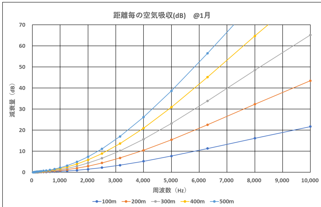
図 305 距離毎の空気吸収による減衰量の試算結果【1月想定】
