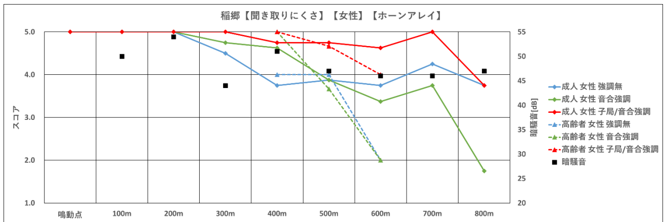
図 173 ホーンアレイ【聞き取りにくさ、稲郷町有地、女性】
