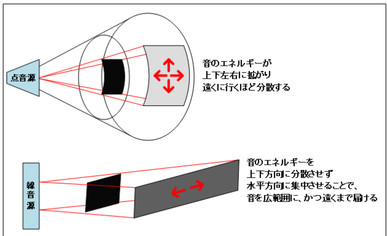
図 9 点音源、線音源の拡がりイメージ
