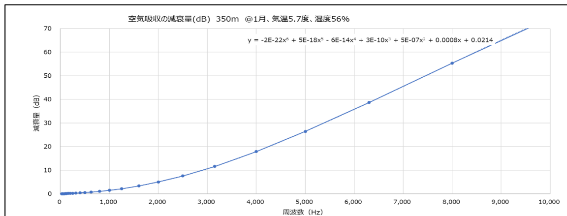
図 47 1 月の空気吸収減衰量
