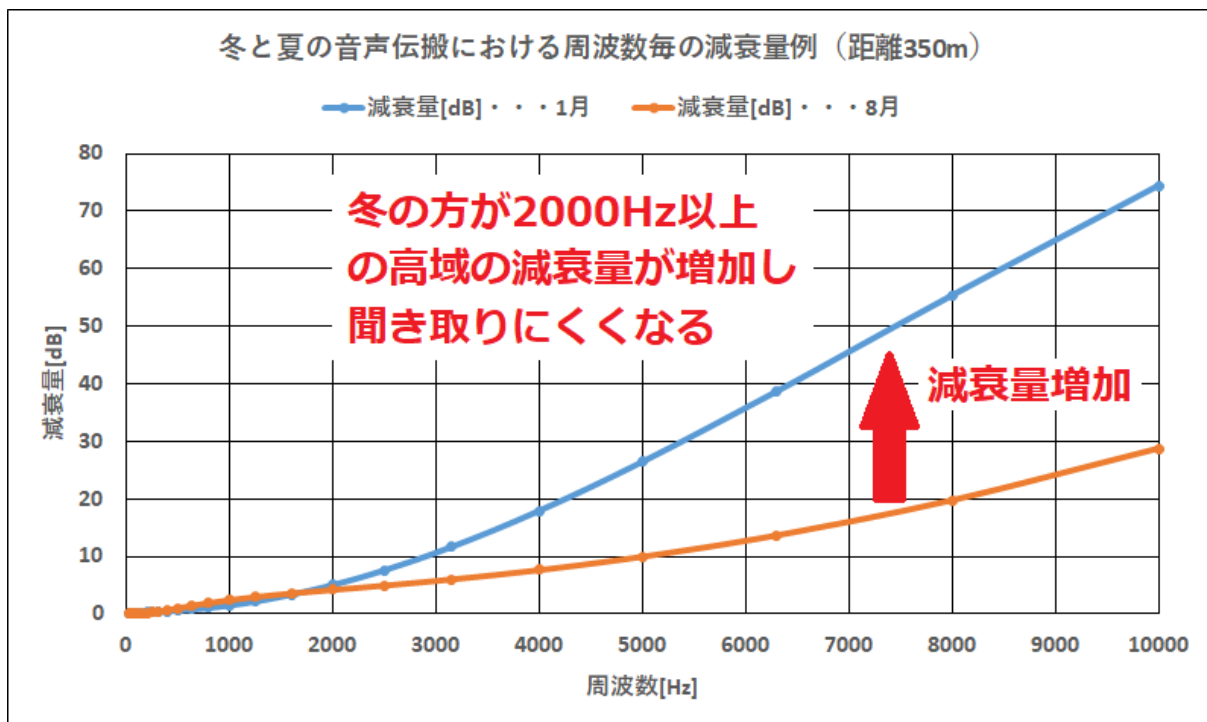
図 41 冬と夏の音声伝搬の周波数特性の試算結果
