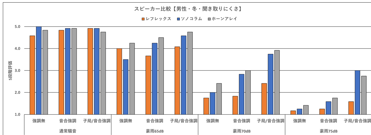
図 63 スピーカー比較【男性・冬・聞き取りにくさ・豪雨】
