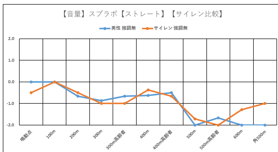
図 266 音声と電子サイレン【音の大きさ、スプラボ、ストレートホーン】
