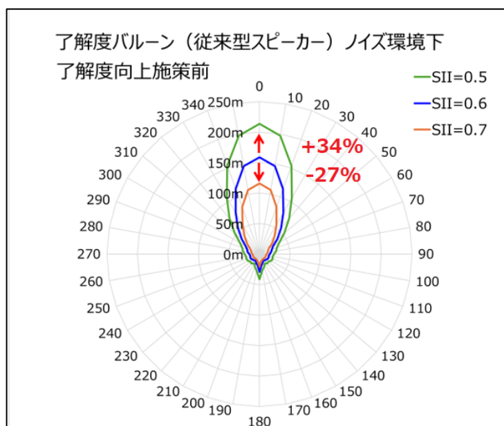
図 40 要求 SII 値と了解度バルーンの関係（例）
