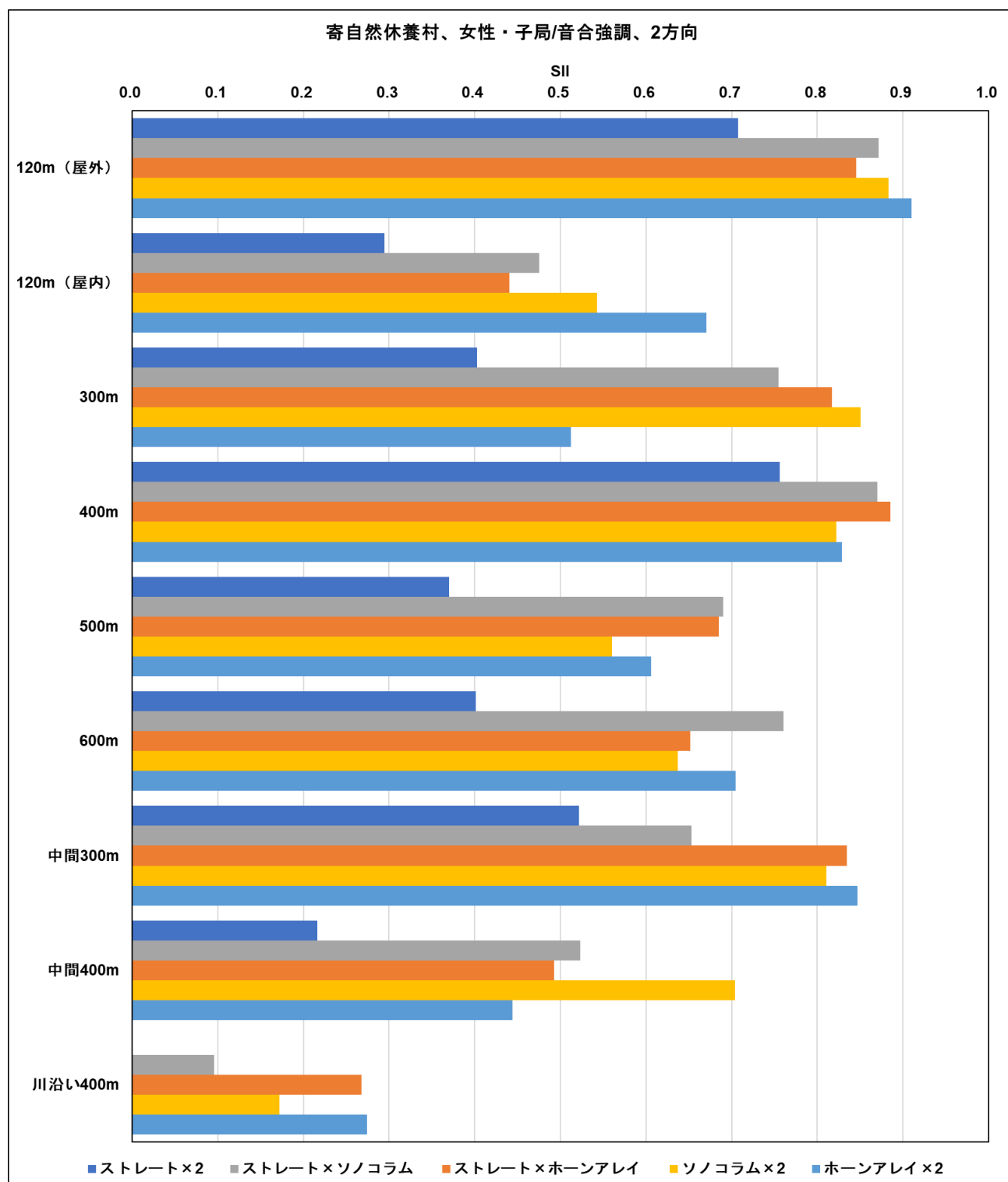
図 283 SII【寄自然休養村 2 方向、女性】
