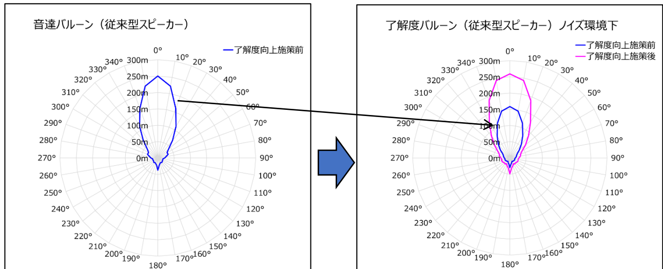
図 301 従来型スピーカーの音達バルーンとノイズ環境下の了解度バルーン計算例
