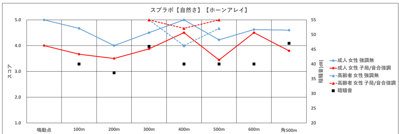
図 182 ホーンアレイ【自然さ、スプラボ、女性】
