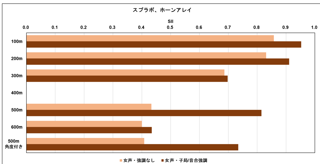
図 272 SII【スプラボ、女性、ホーンアレイ】
