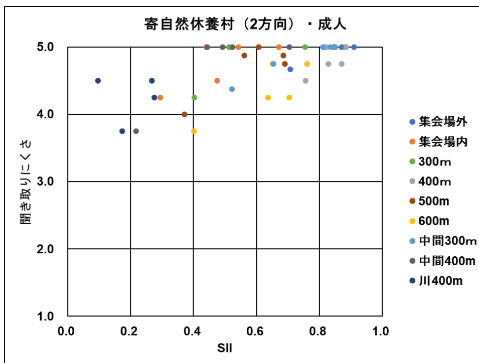
図 293 SII と聞き取りにくさの関係【寄自然休養村 2 方向、成人】
