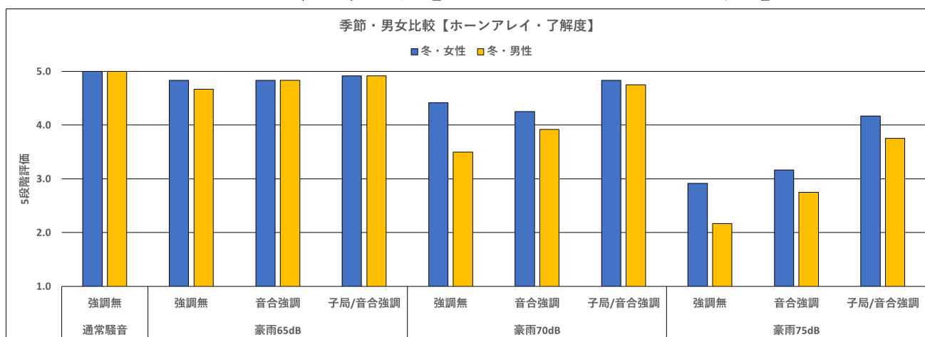
図 74 話者（男女）比較【ホーンアレイ・冬・了解度・豪雨】
