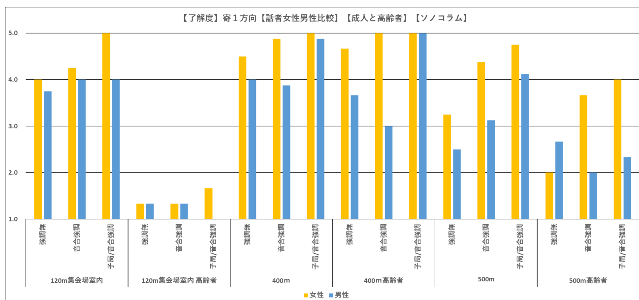
図 235 話者（男女）の違い【了解度、寄自然休養村、成人・高齢者、ソノコラム】
