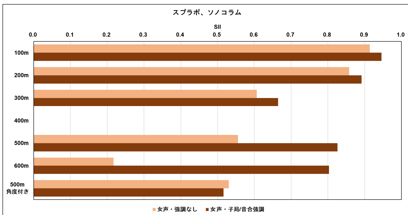
図 271 SII【スプラボ、女性、ソノコラム】
