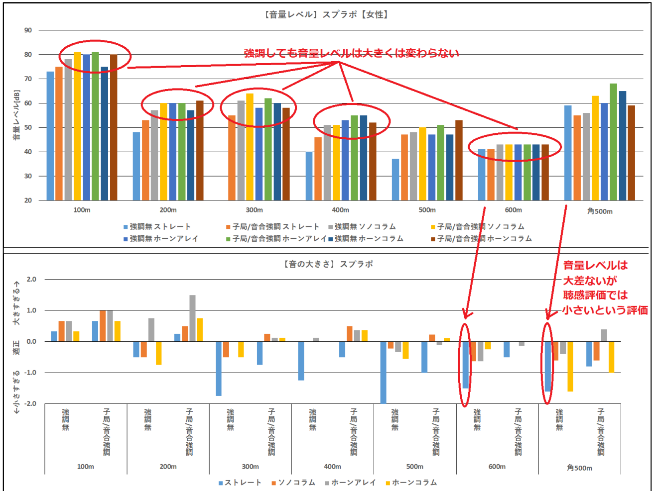
図 26 音量レベルと音の大きさ評価の関係【スプラボ、話者女性】
