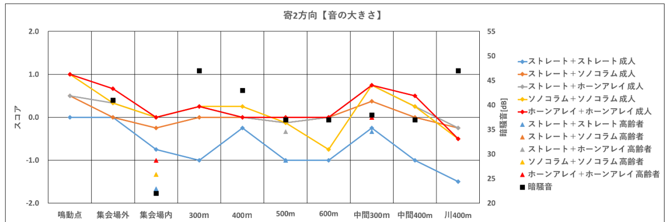
図 259 二方向鳴動【音の大きさ、寄自然休養村、女性、成人・高齢者、全スピーカー】
