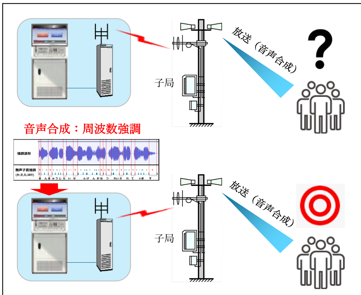
図 312 音声合成の周波数強調導入イメージ
