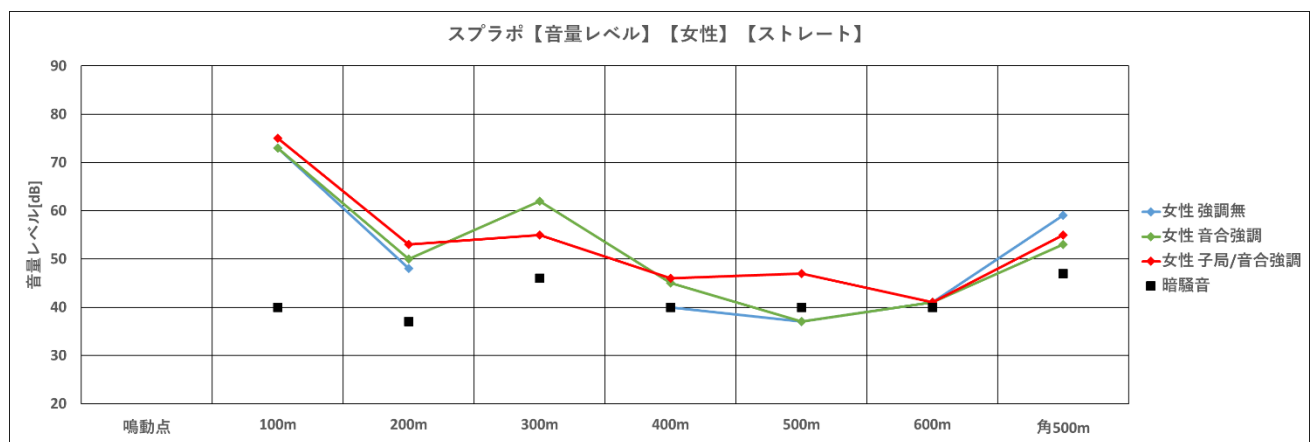
図 194 ストレートホーン【音量レベル、スプラポ、女性】
