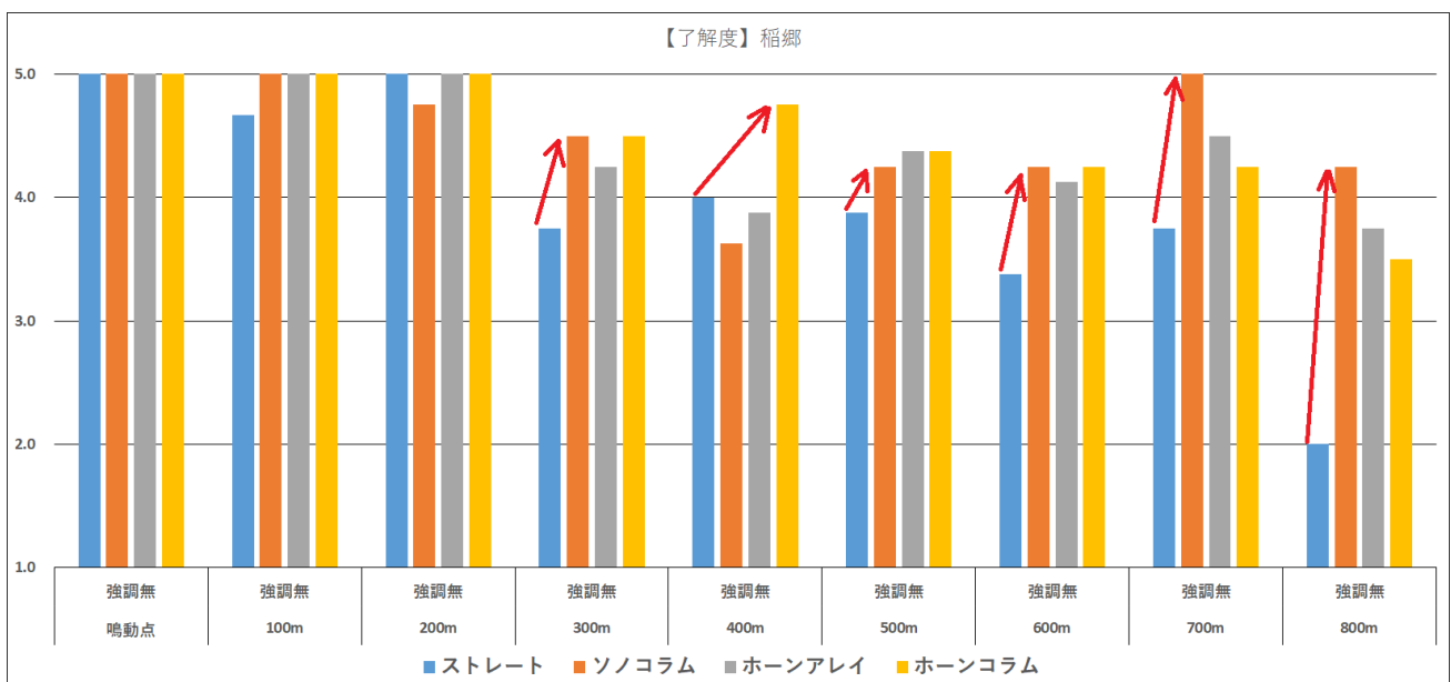
図 28 スピーカー比較【了解度、稲郷、話者女性、音声改善施策無しで比較】
