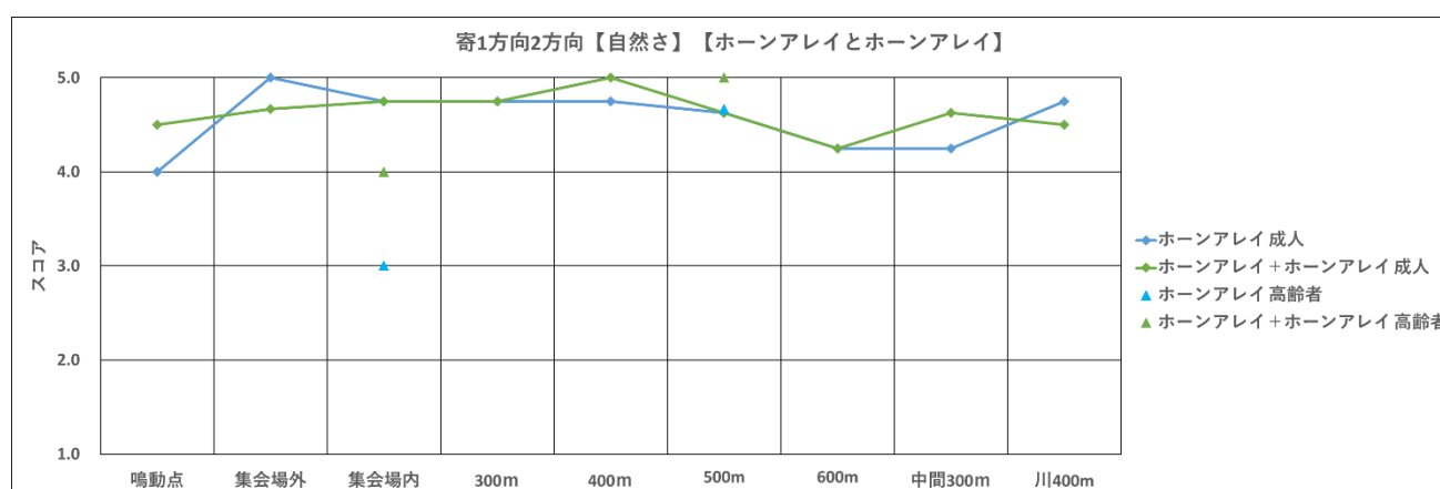
図 258 一方向二方向比較【自然さ、寄自然休養村、女性、成人・高齢者、ホーンアレイ】
