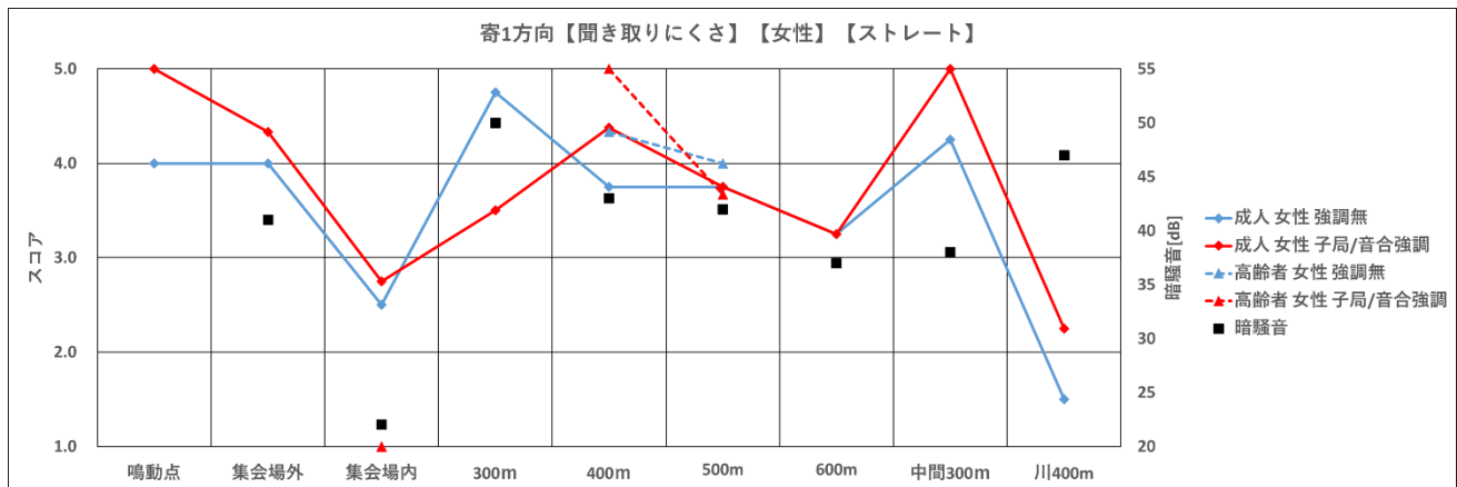
図 176 ストレートホーン【聞き取りにくさ、寄自然休養村、女性】
