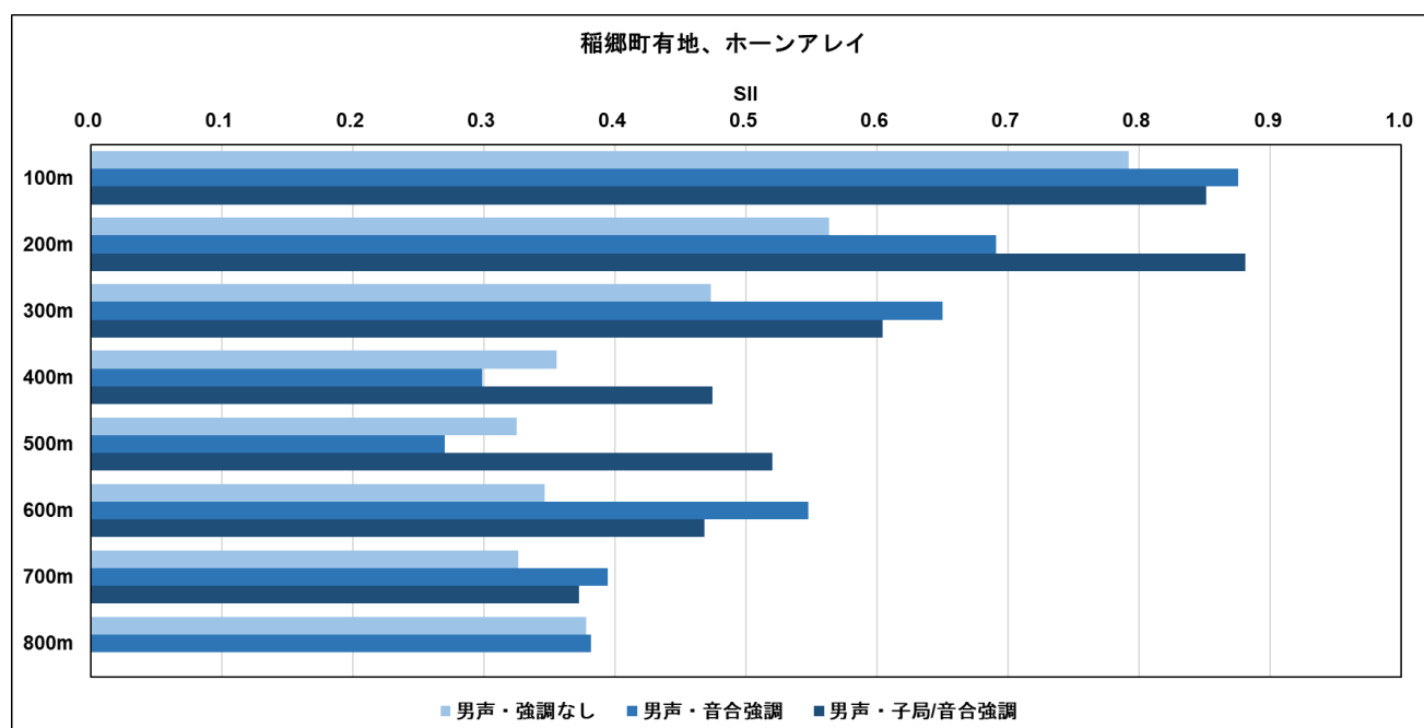
図 277 SII【稲郷町有地、男性、ホーンアレイ】
