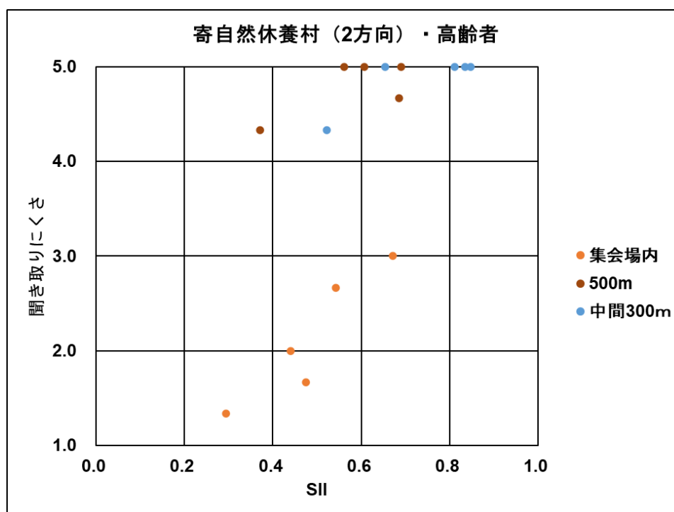
図 294 SII と聞き取りにくさの関係【寄自然休養村 2 方向、高齢者】
