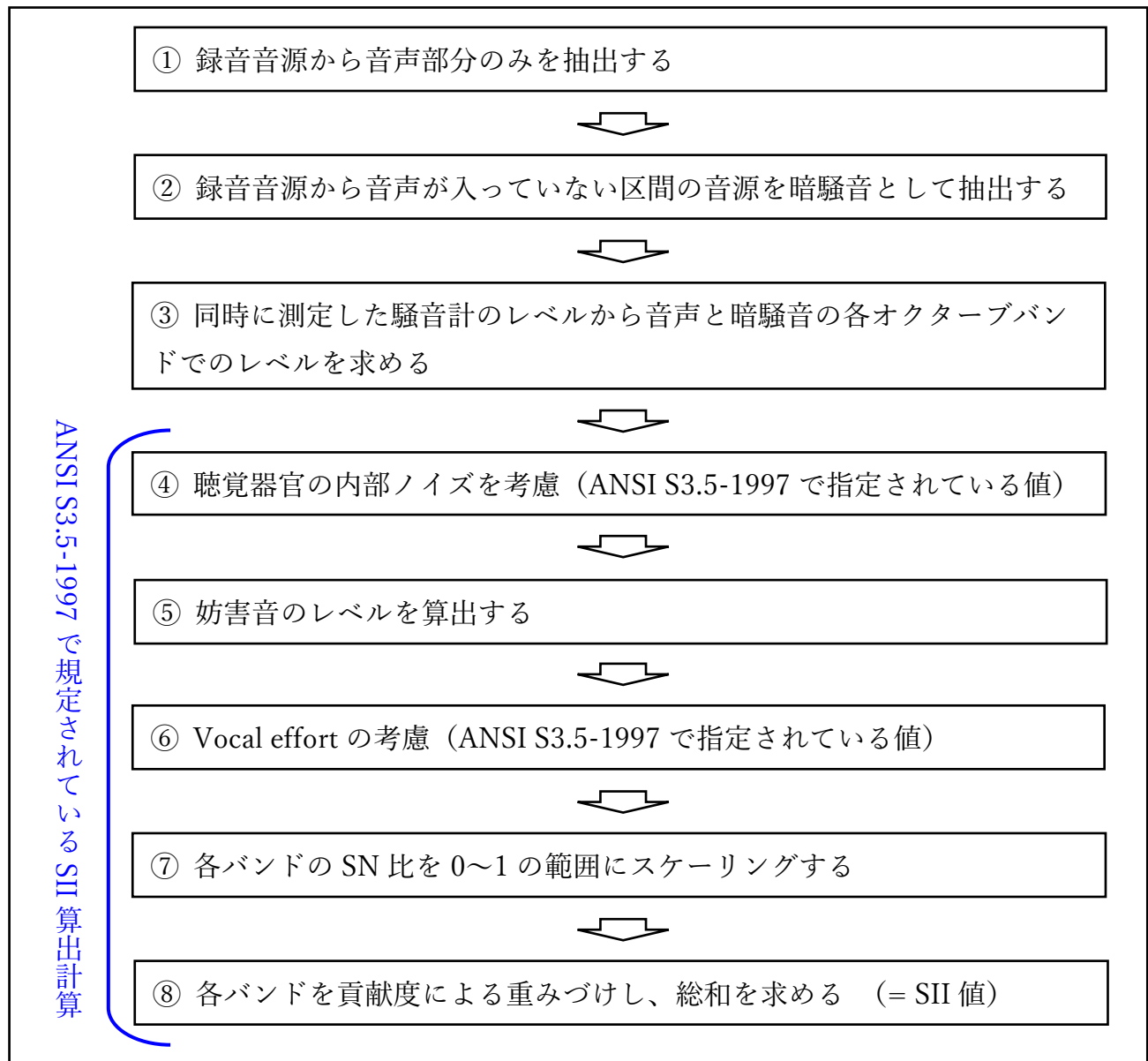
図 116 放送音声からの SII 計算手順
