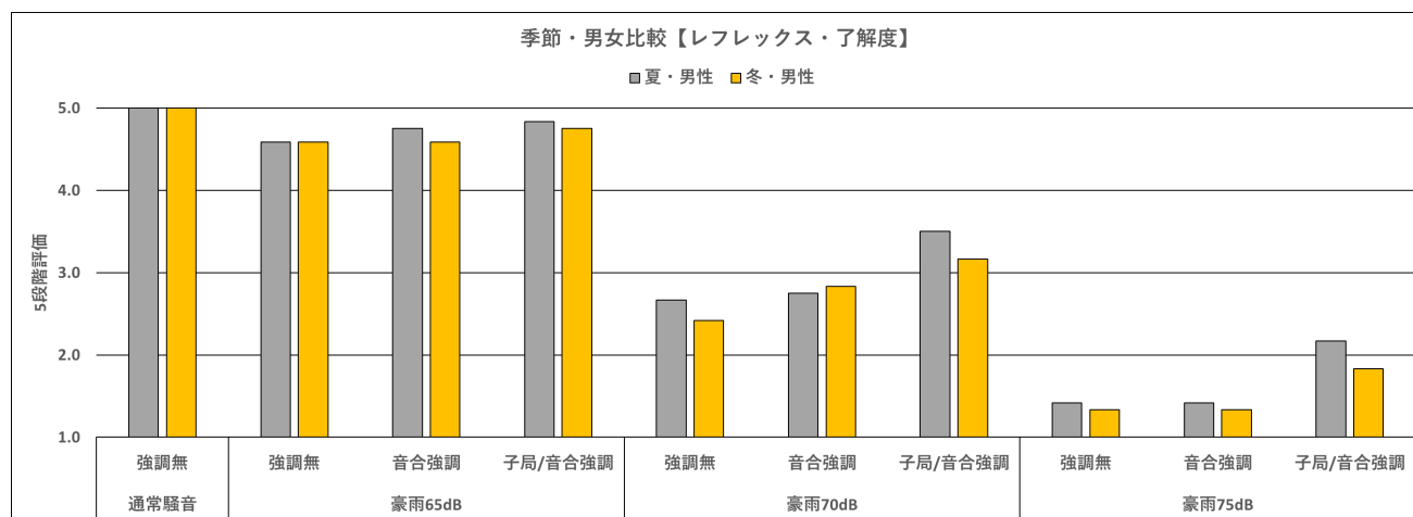
図 90 季節（夏冬）比較【レフレックス・男性・了解度・豪雨】
