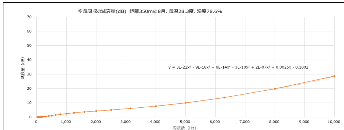
図 48 8 月の空気吸収減衰量
