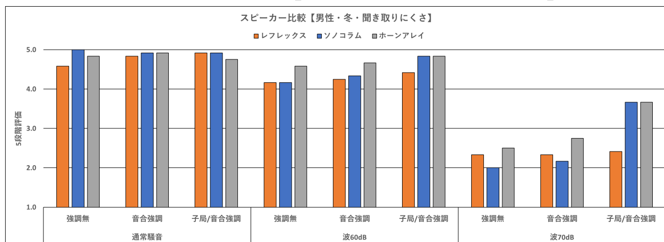
図 64 スピーカー比較【男性・冬・聞き取りにくさ・波】
