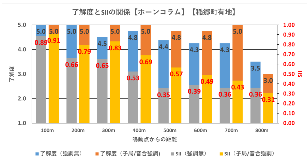
図 36 了解度と SII の関係（稲郷町有地、ホーンコラム）
