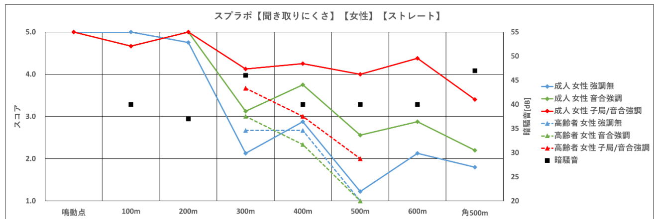
図 166 ストレートホーン【聞き取りにくさ、スプラゴ、女性】
