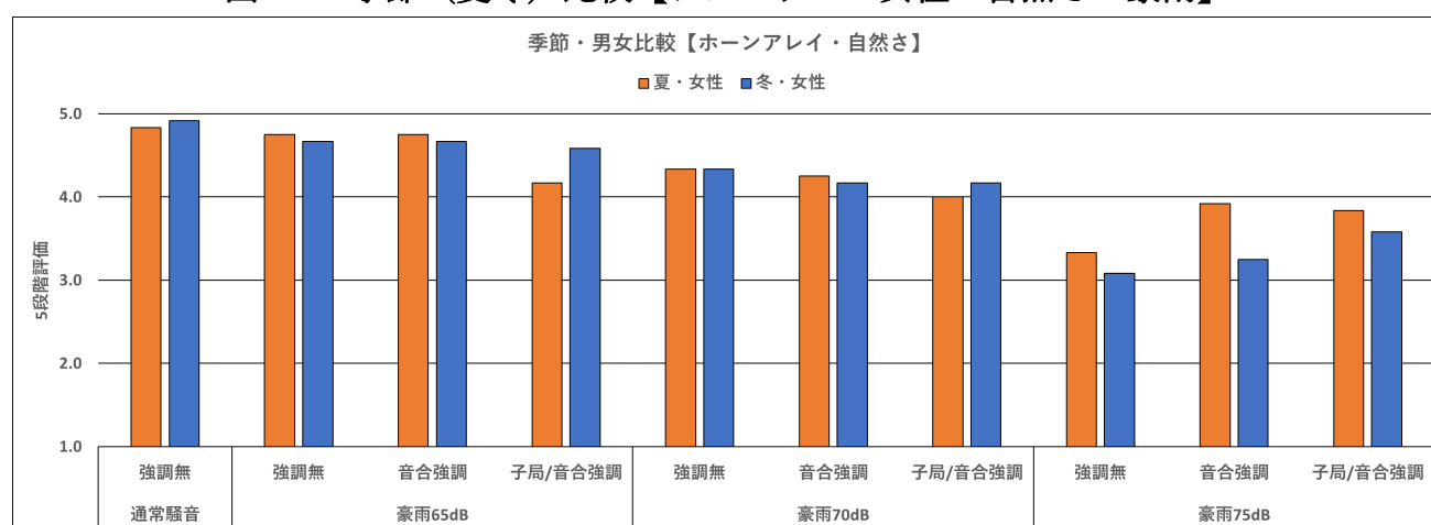
図 95 季節（夏冬）比較【ホーンアレイ・女性・自然さ・豪雨】
