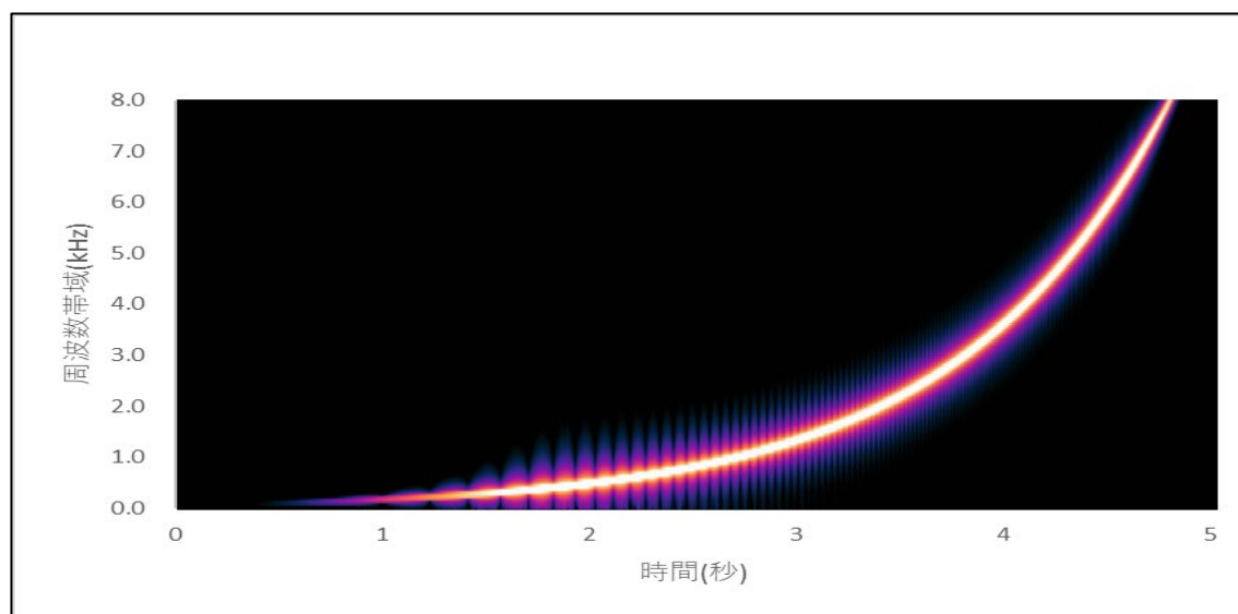
図 114 Swept-Sine 信号
