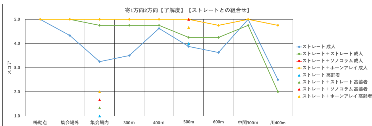
図 246 一方向二方向比較【了解度、寄自然休養村、女性、成人・高齢者、ストレート】
