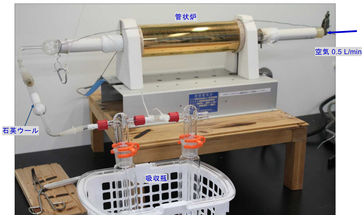
写真 3 加熱試験の様子
