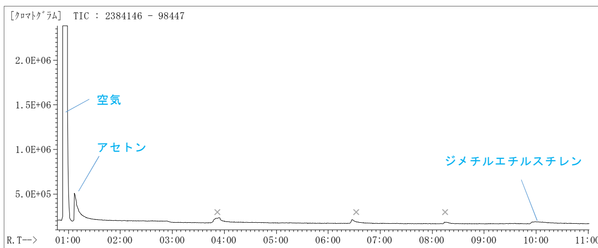
図 1 加熱発生ガスの GCMS クロマトグラム（トータルイオンクロマト）
