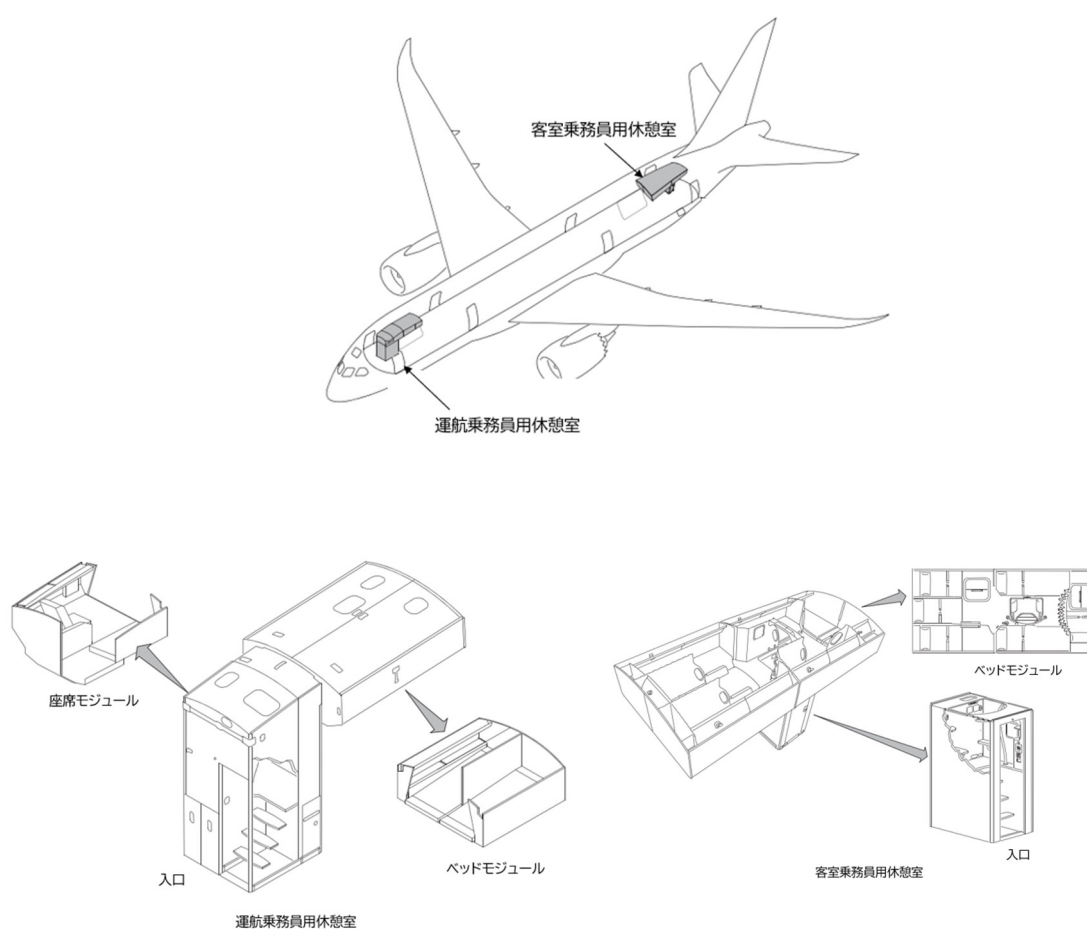
図 7.26. 乗務員用の休憩室設置場所
