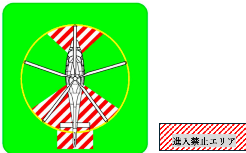
図 7.40. ローター回転時の危険区域
