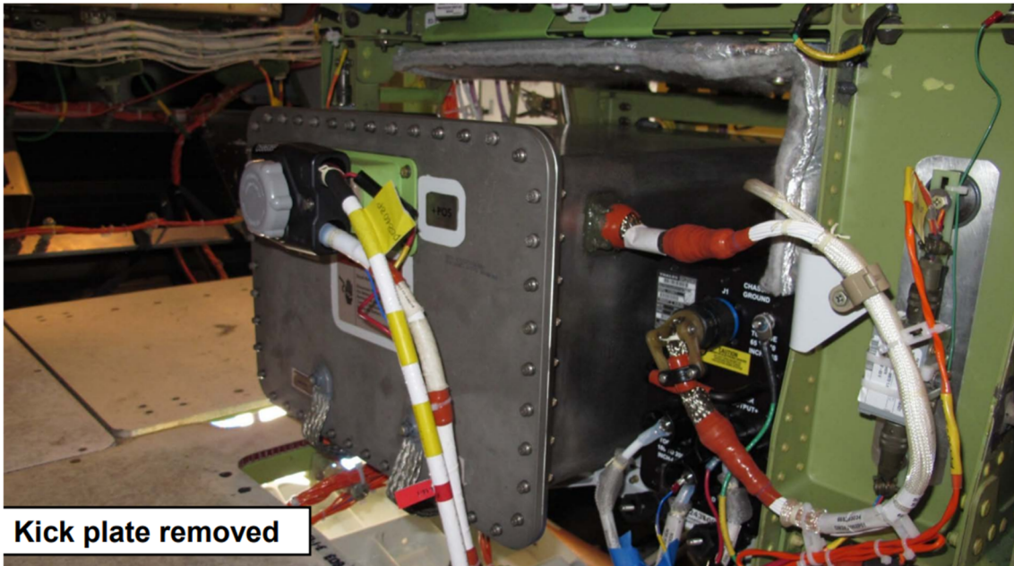
図 7.15. バッテリー筐体(エンクロージャー)
