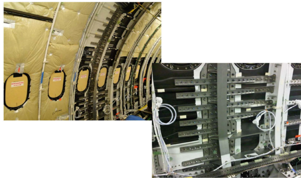
図 7.22. 補強されている箇所
