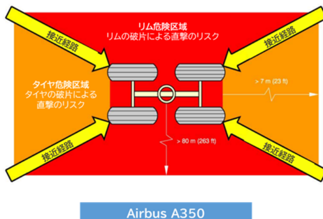
図 7.8 航空機のタイヤ・リム危険区域と接近経路(Airbus 社の例 2)
