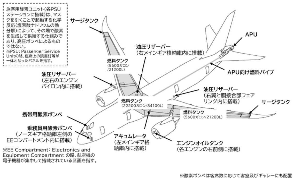
図 2.4. 燃料・油圧系統及び酸素ボンベ概略図(B787)
