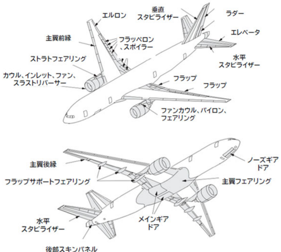
図 2.7. アルミニウム合金主体(B777)の複合材使用箇所例
