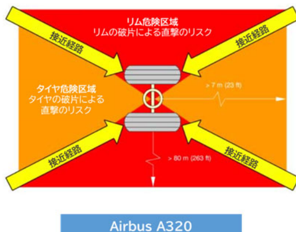
図 7.7 航空機のタイヤ・リム危険区域と接近経路(Airbus 社の例 1)
