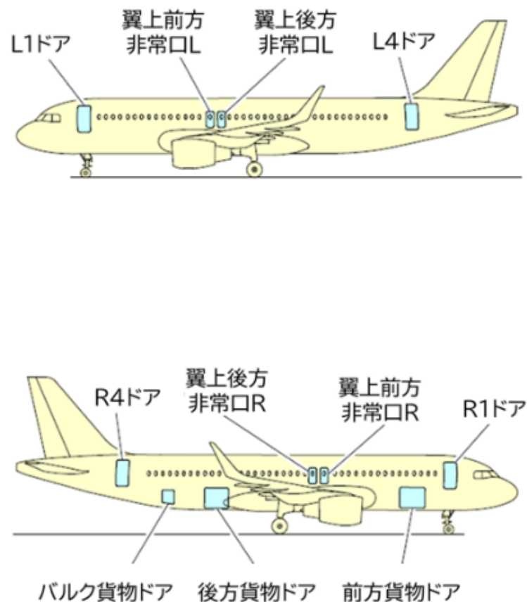
図 7.17. 航空機の主要なドアの位置(例 A320)
