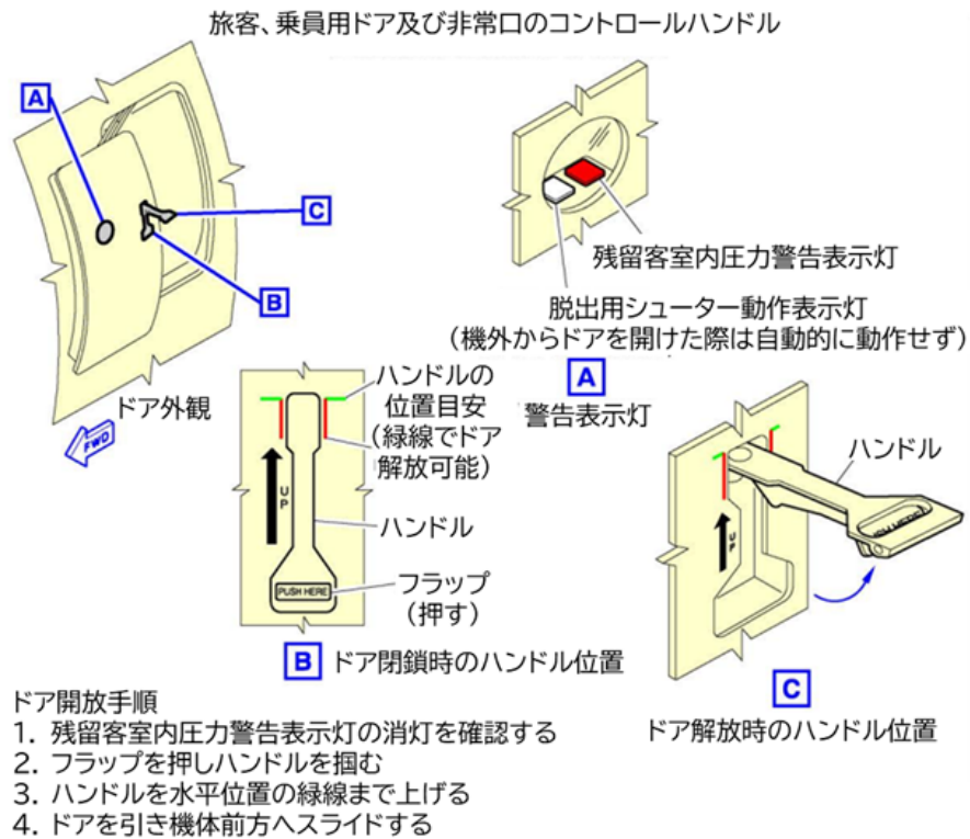
図 7.18. ドアの開放要領(例 A320)
