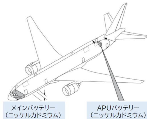
図 2.5. B777 バッテリー配置概略図
