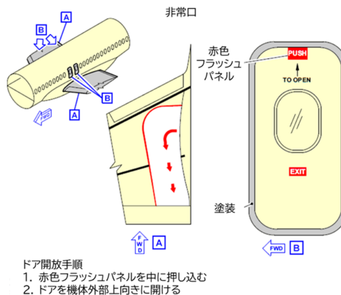
図 7.19. ドアの開放要領(例 A320 非常口)
