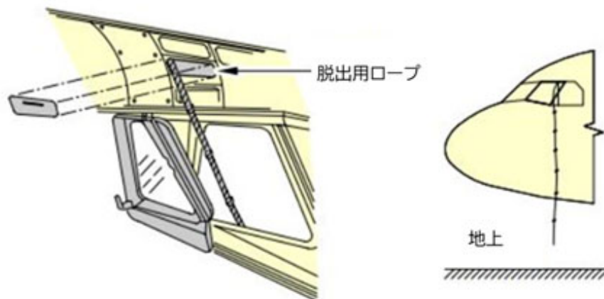
図 2.10. 脱出用スライド及び脱出用ロープ展開例②(A320)
