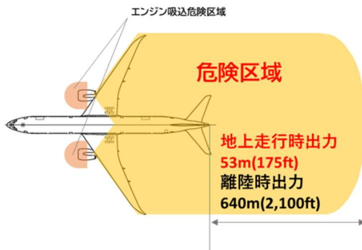
図 7.4. 航空機エンジン稼働時の危険区域(離隔範囲) (例:B787(GE エンジン)の場合)
