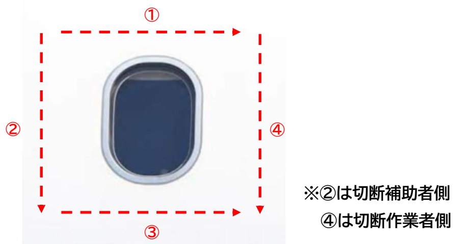
図 7.24. 切断する順番
