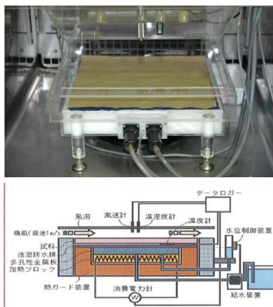
【図 4-9 試験装置イメージ図】
