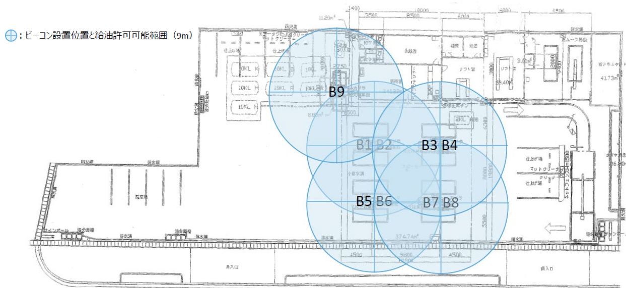
図11 ビーコンによる給油許可等の範囲設置位置（小規模施設）
