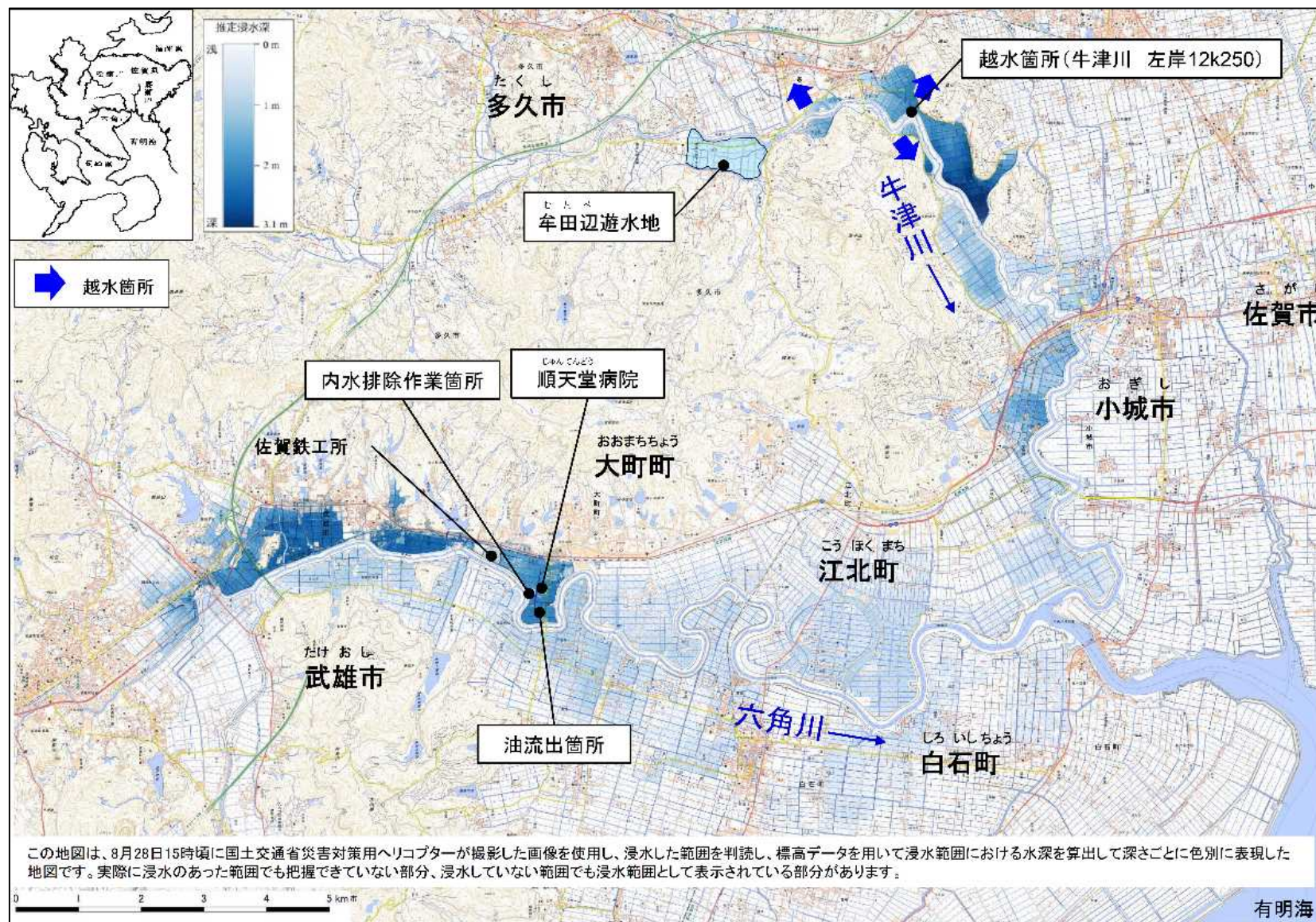
六角川水系における浸水推定段彩図
