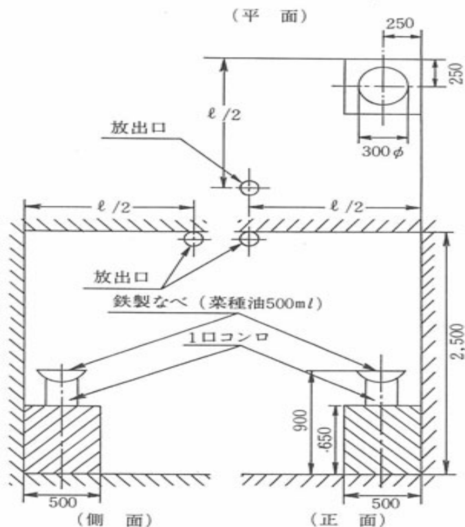
別図 3 第 3 消火試験図 [単位：ミリメートル]
