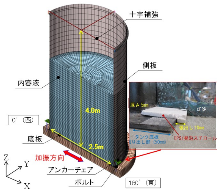
図 3-2 対策工法 1 底板張出部上 緩衝材設置イメージ
