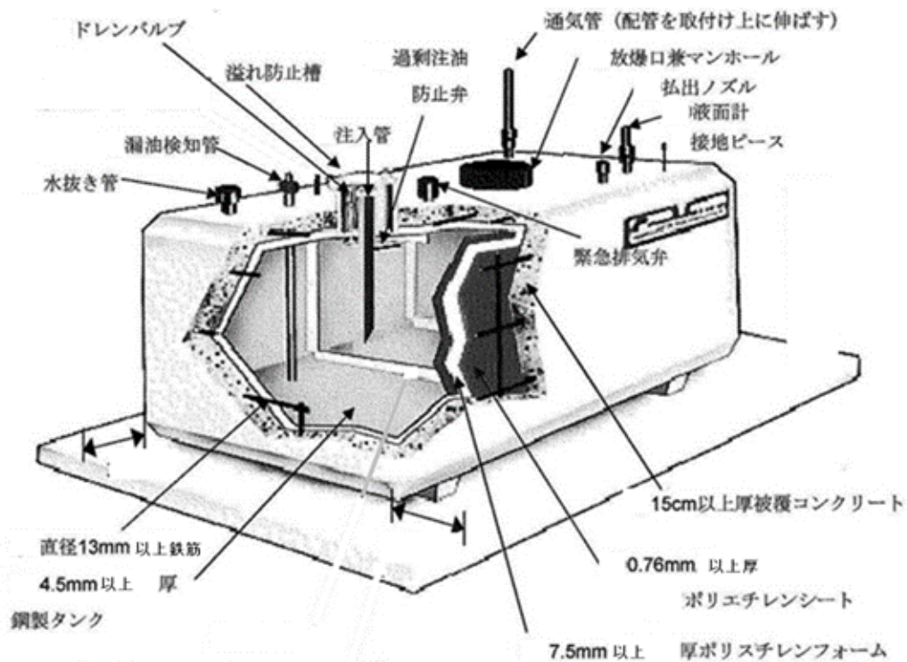
図 2-27 コンクリート被覆型タンクの構造
