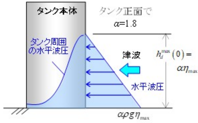
図3-7 タンク本体に作用する津波波圧分布
