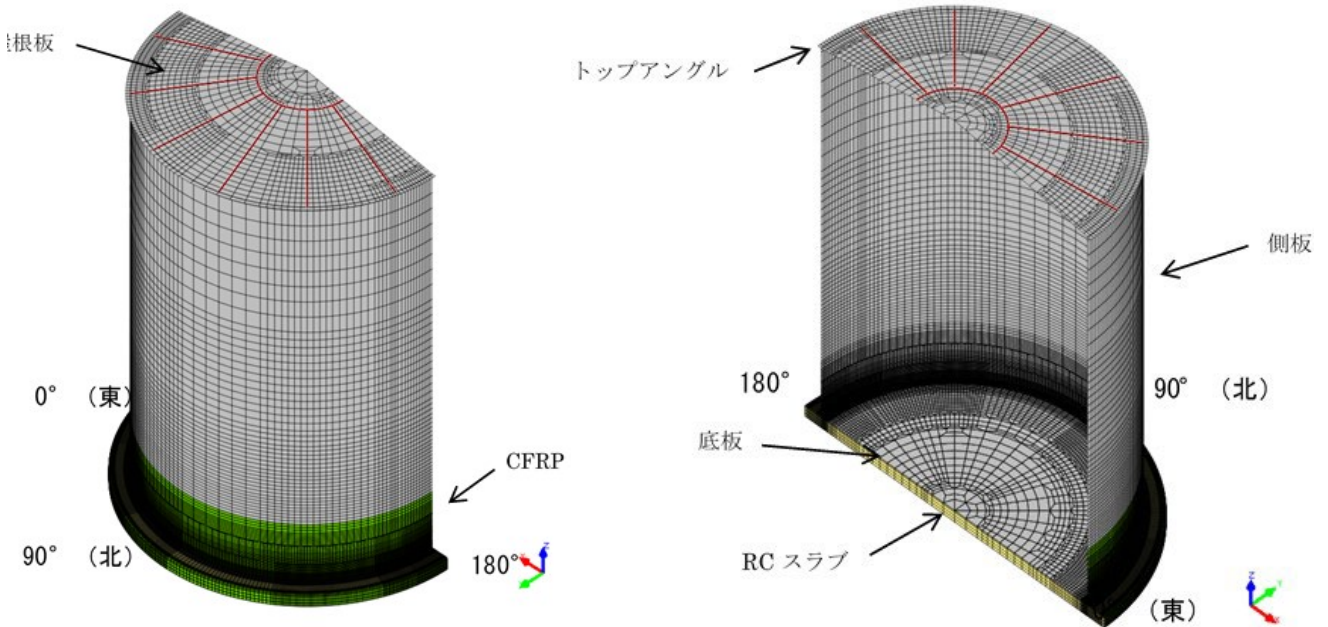
図 3-5.1 100 kL 級タンク 対策工法 1 の解析モデル全体図
