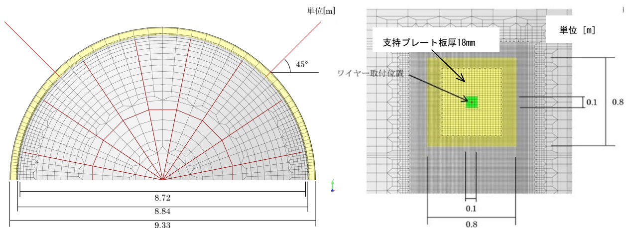
図3-10.2 500 kL 級タンク 対策工法2の解析モデル上面図とワイヤー支持部拡大図
