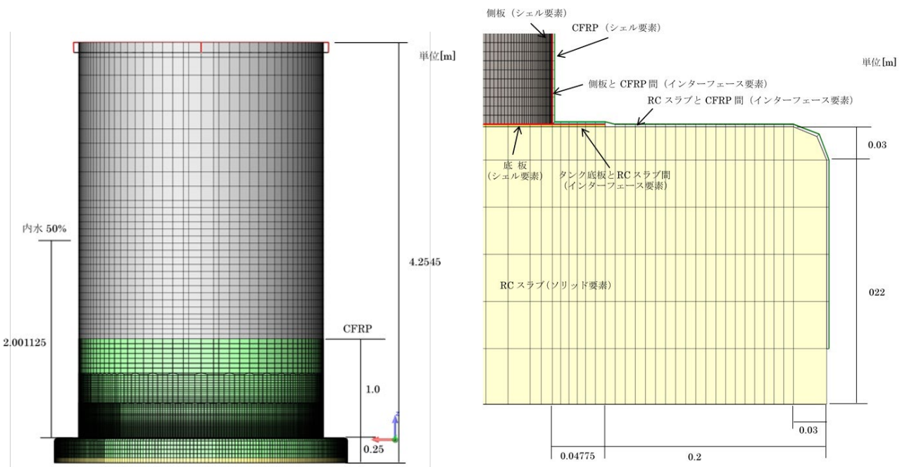
図 3-4.2 20 kL 級タンク 対策工法 1 の解析モデル正面図と底板と基礎拡大図
