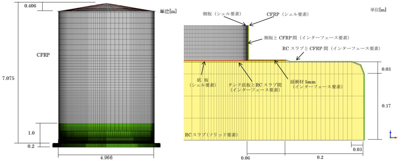
図 3-5.2 100 kL 級タンク 対策工法 1 の解析モデル正面図と底板と基礎拡大図
