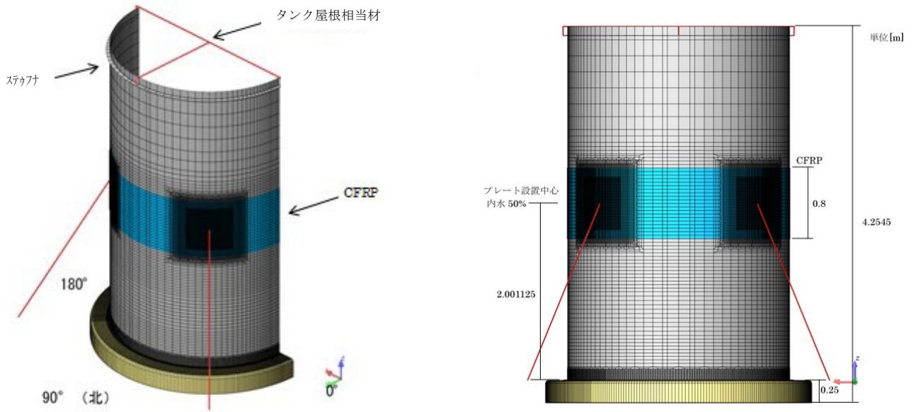
図 3-8.1 20 kL 級タンク 対策工法 2 の解析モデル全体図
