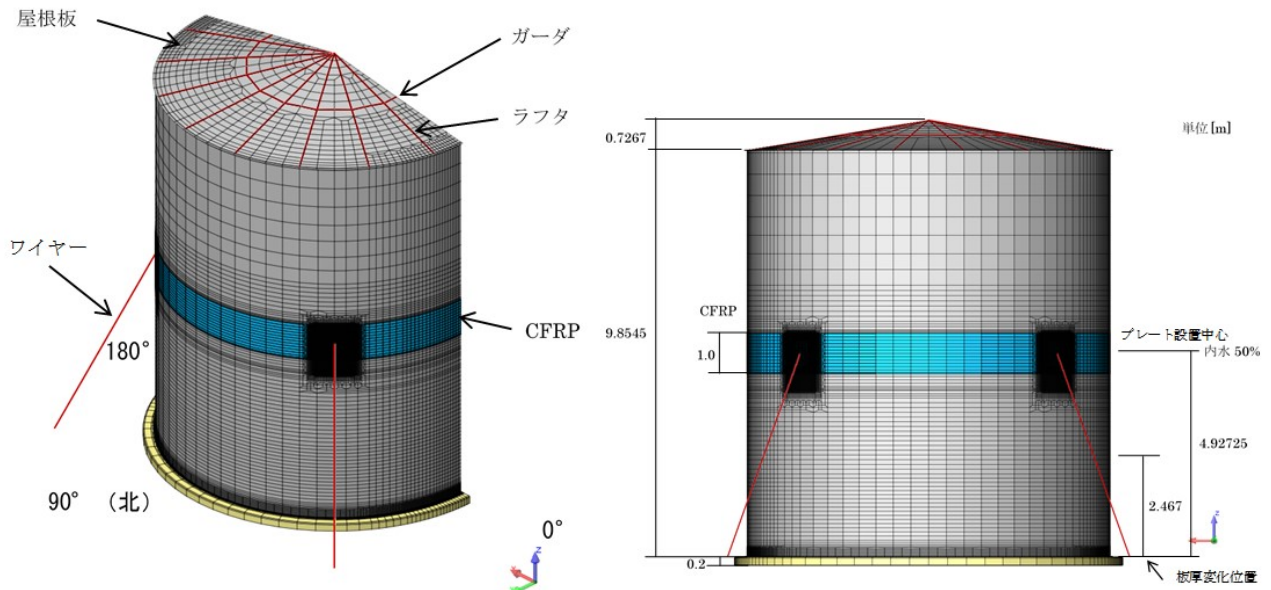
図3-10.1 500 kL 級タンク 対策工法2の解析モデル全体図
