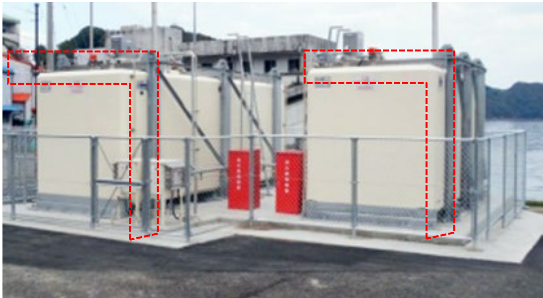
図 2-30 津波対策型コンクリート被覆型タンクの例 (メーカーホームページ http://convault.jp/ より)
