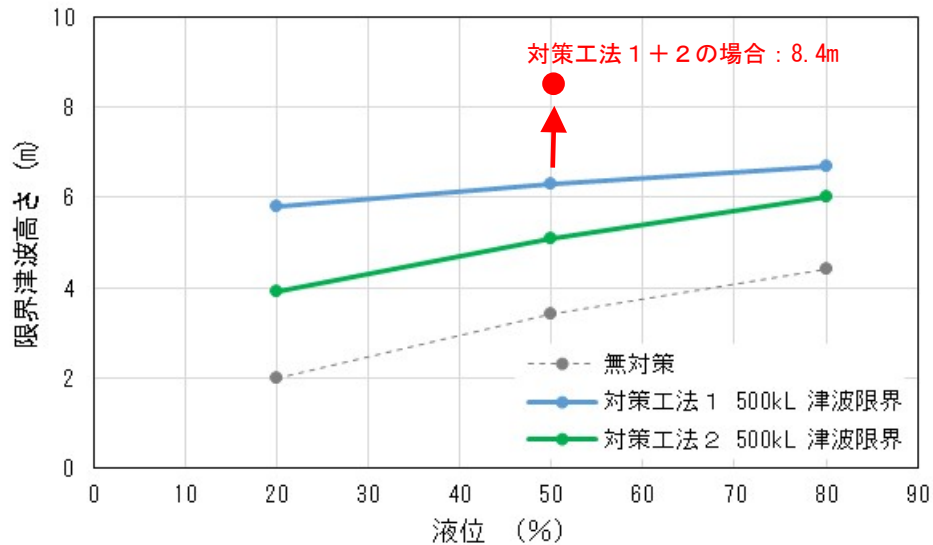
図3-13 対策工法による津波限界水位の比較
