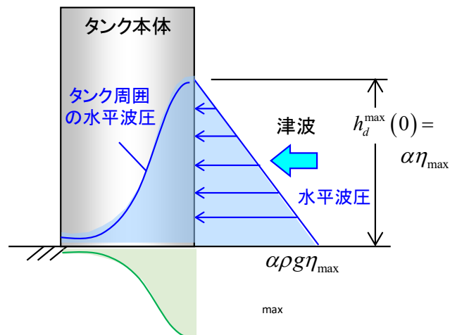
図3-11 タンク本体に作用する津波波圧分布
