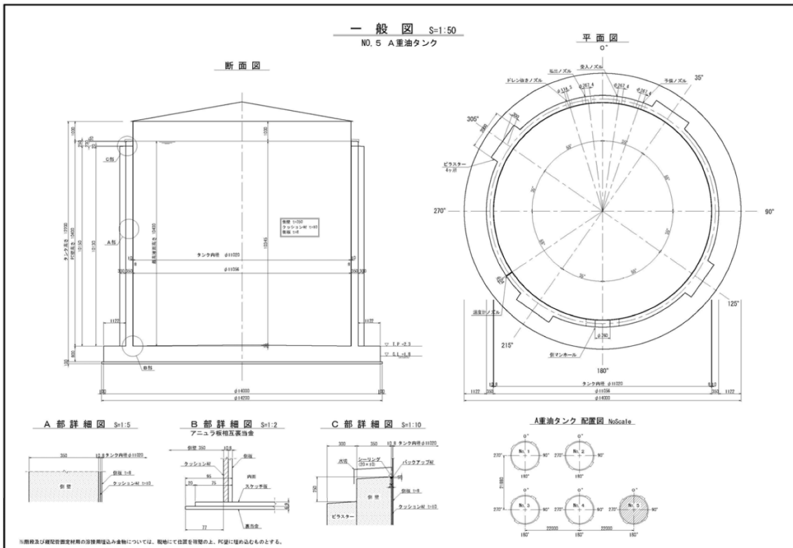
図 2-25 タンク仕様
