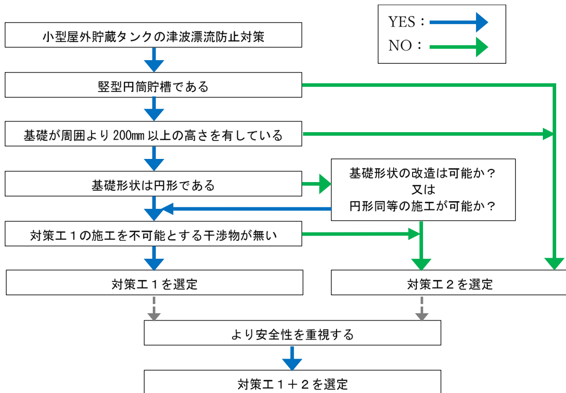
図 3-14 対策工法の選定フロー
