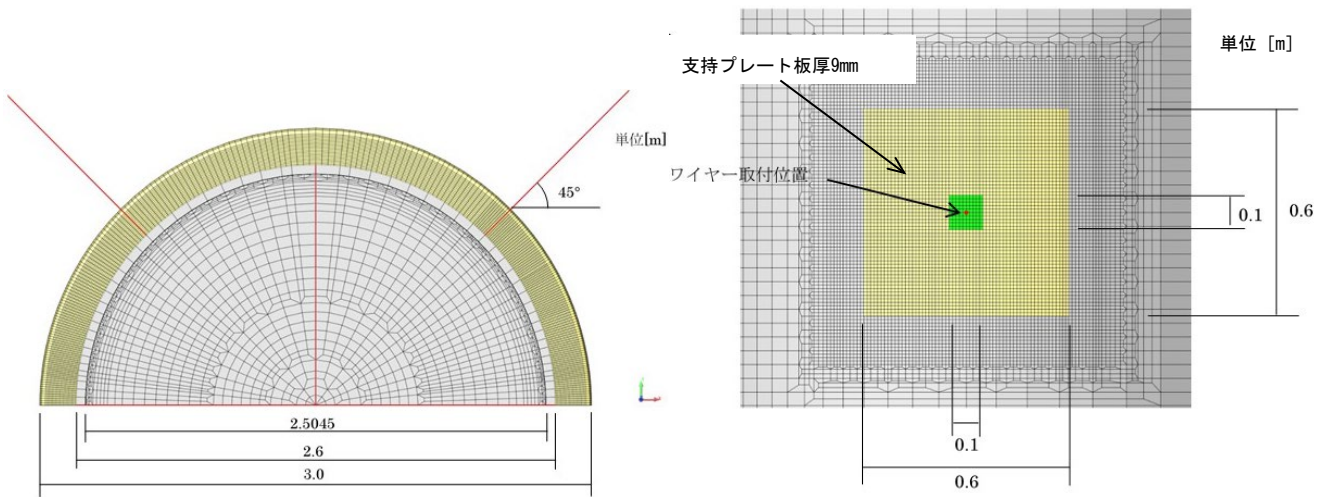
図 3-8.2 20 kL 級タンク 対策工法 2 の解析モデル上面図とワイヤー支持部拡大図
