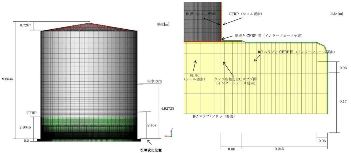
図 3-6.2 500 kL 級タンク 対策工法 1 の解析モデル正面図と底板と基礎拡大図
