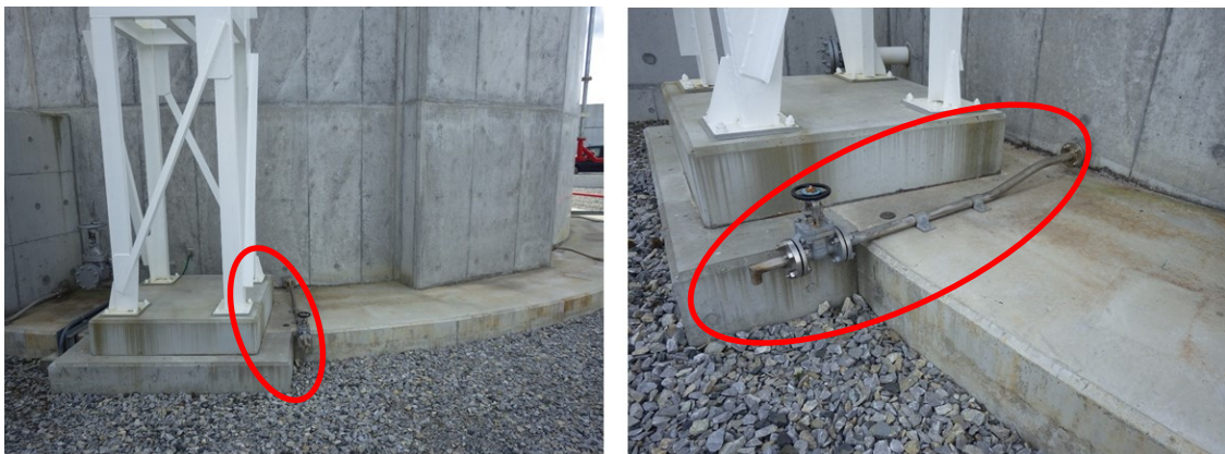
図 2-23 タンク本体とPC壁間の排水管とバルブ
