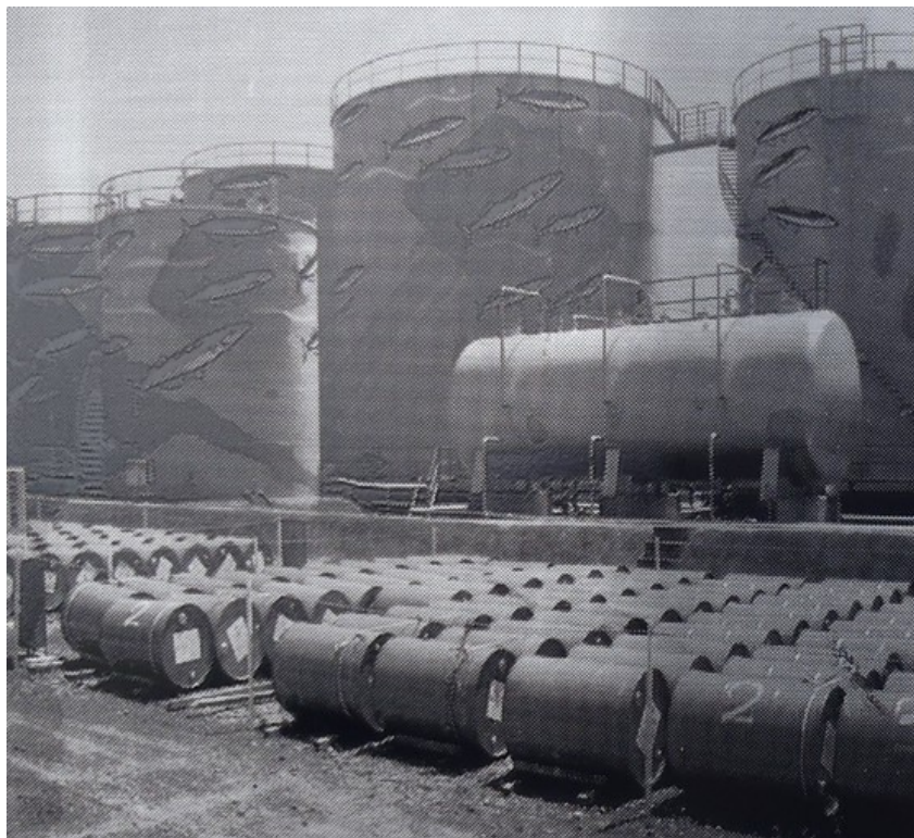
図2-21 2011年東北地方太平洋沖地震前の同油槽所
