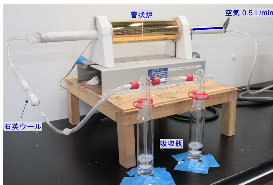
写真 5 加熱試験の様子
