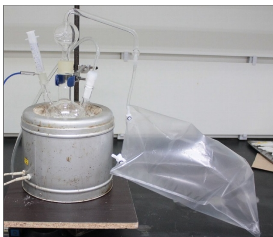
写真3 水添加試験の様子 (バッグ捕集を用いた条件)
