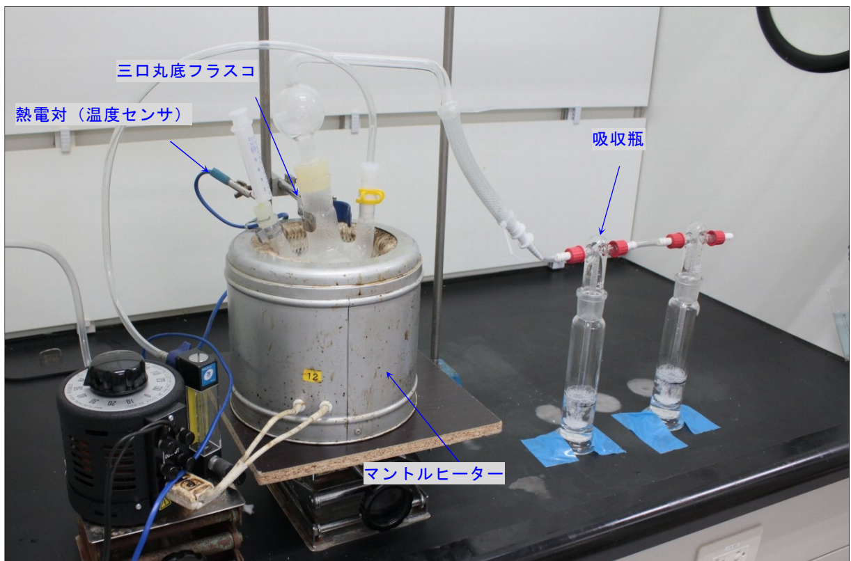
写真 2 水添加試験の様子（吸収瓶を用いた条件）
