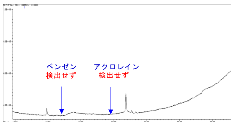
図4 ベンゼン・アクロレイン-GCMS
