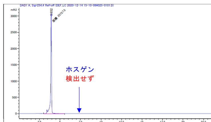
図3 ホスゲン-HPLC
