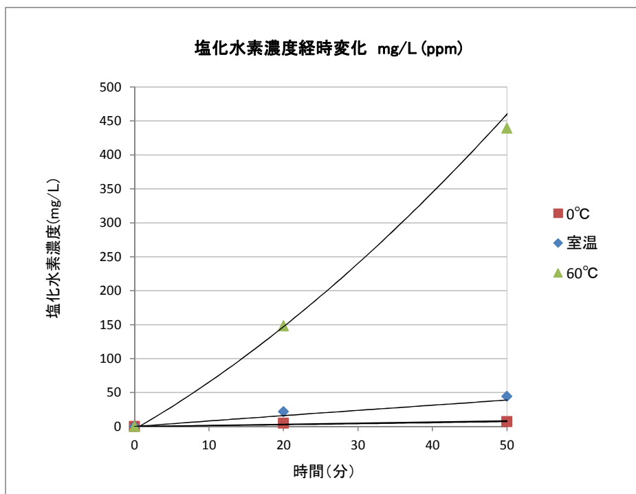
図2 水溶液中の塩化水素量の経時変化
