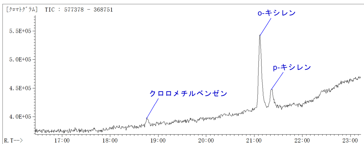
図1 GCMS クロマトグラム（濃度は算出せず）
