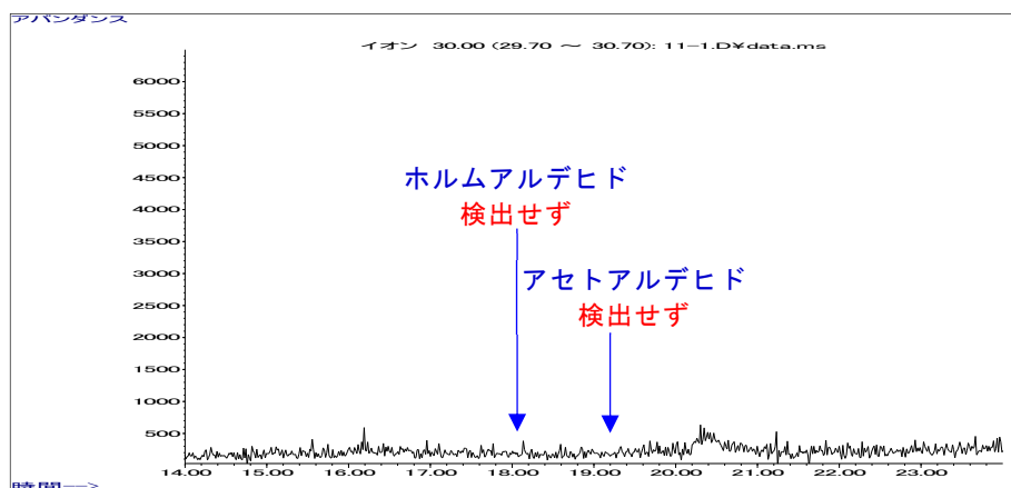
図5 ベンゼン・アクロレイン-GCMS
