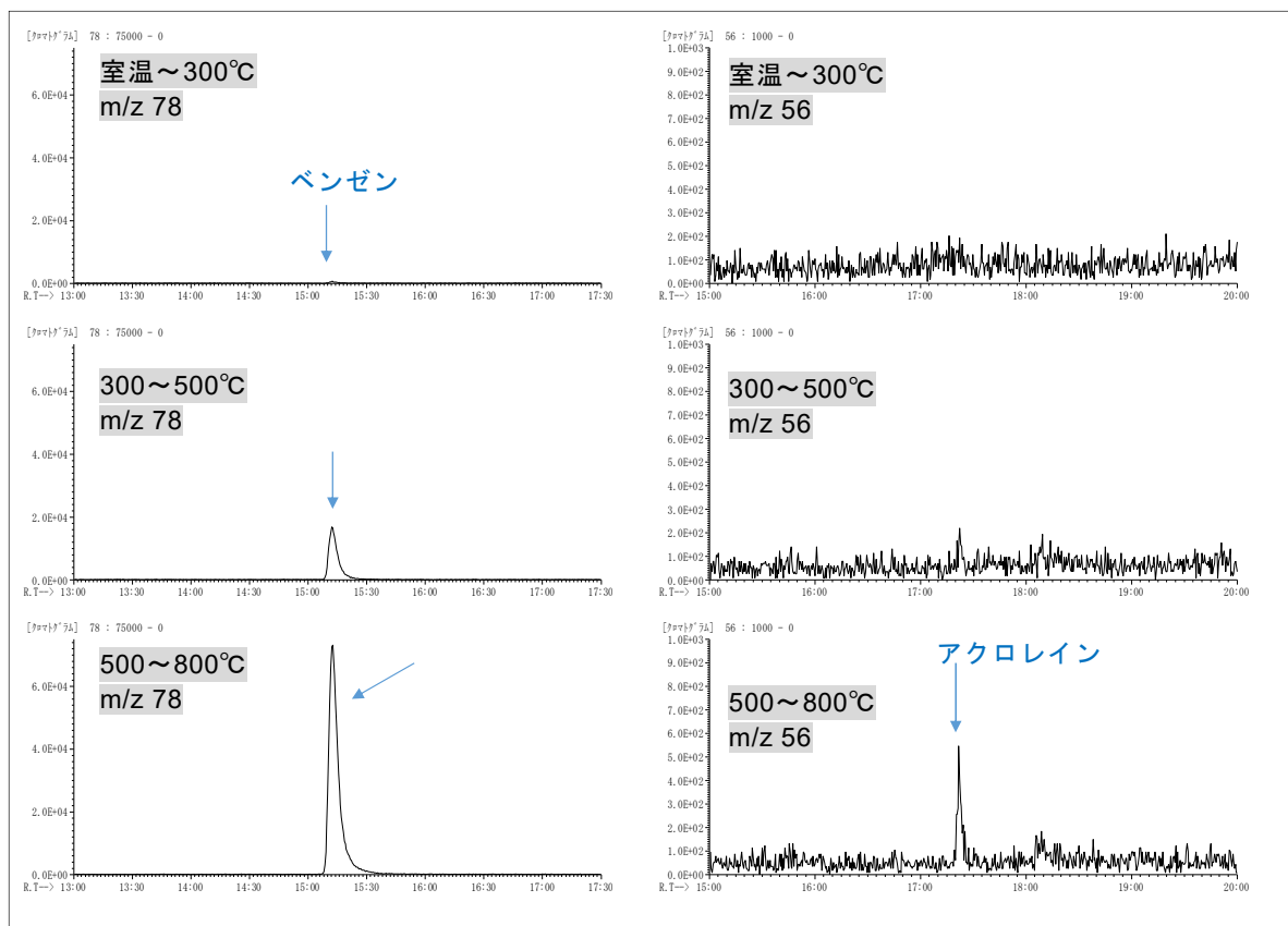
図5 ベンゼン・アクロレイン
