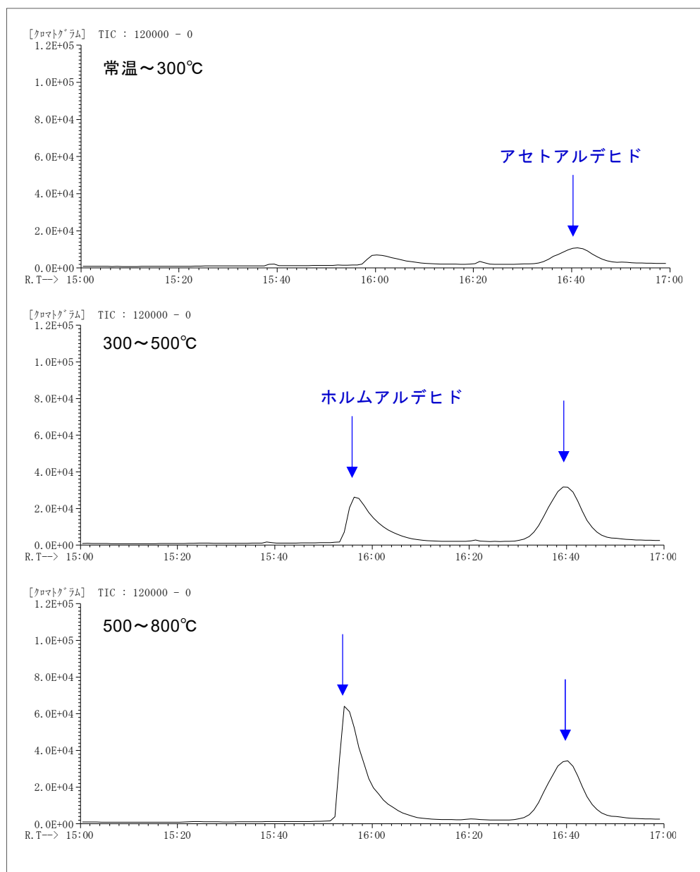
図3 アルデヒド類
