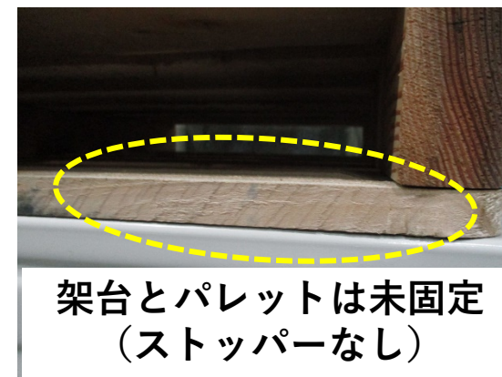
No.06 架台とパレットの固定状況
